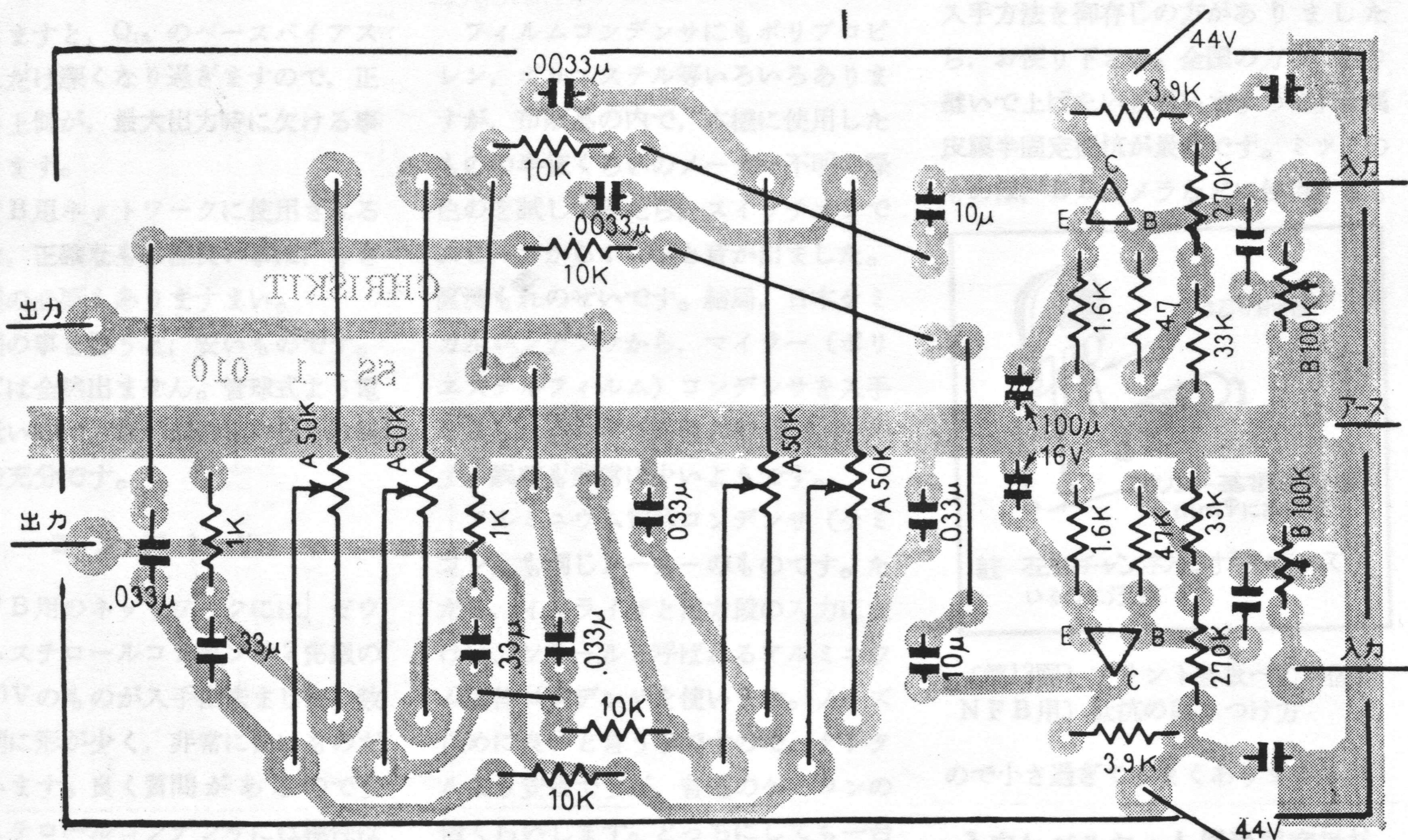
(a) トーンコントロール段のパターン図
