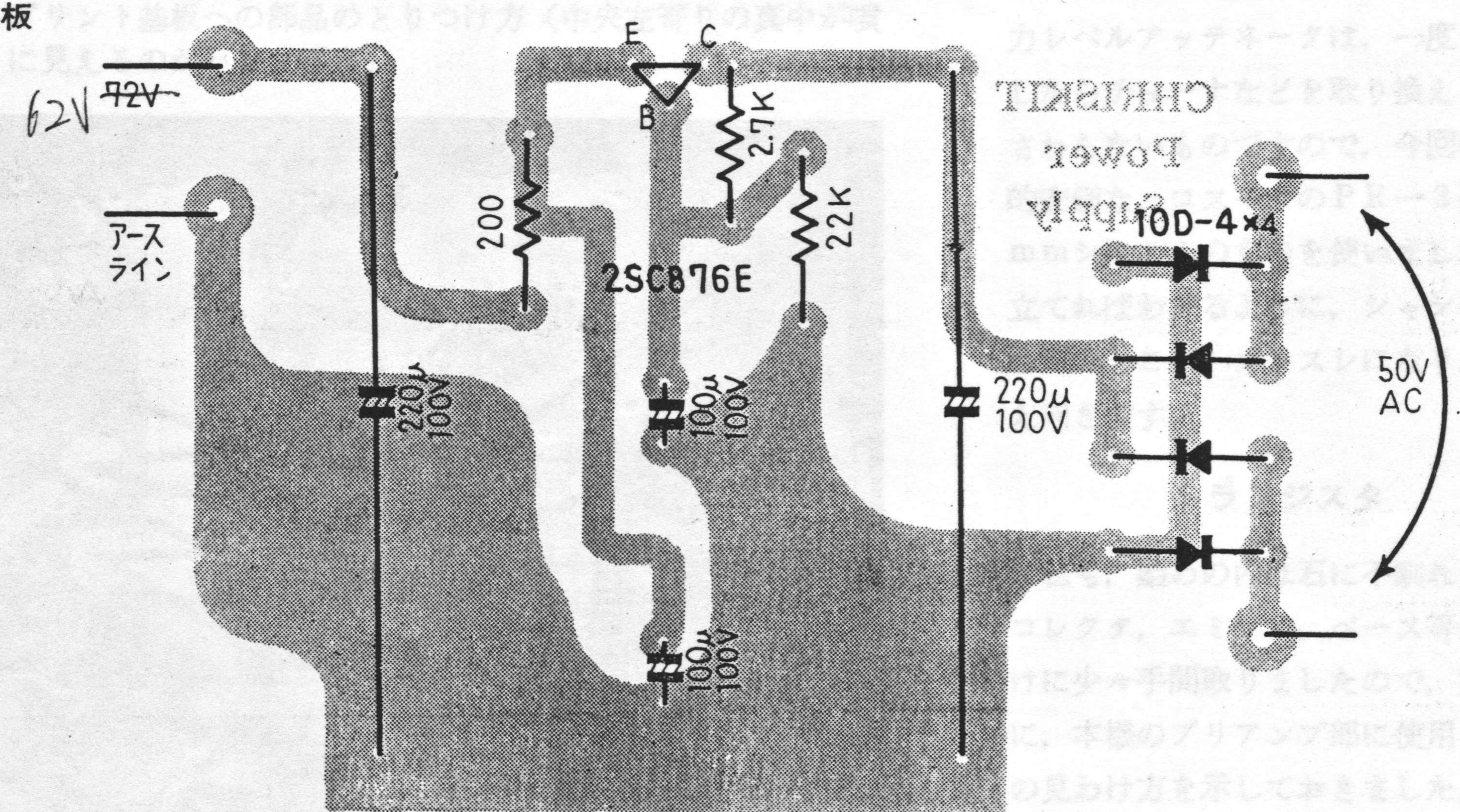
(b) 電源部のパターン図
