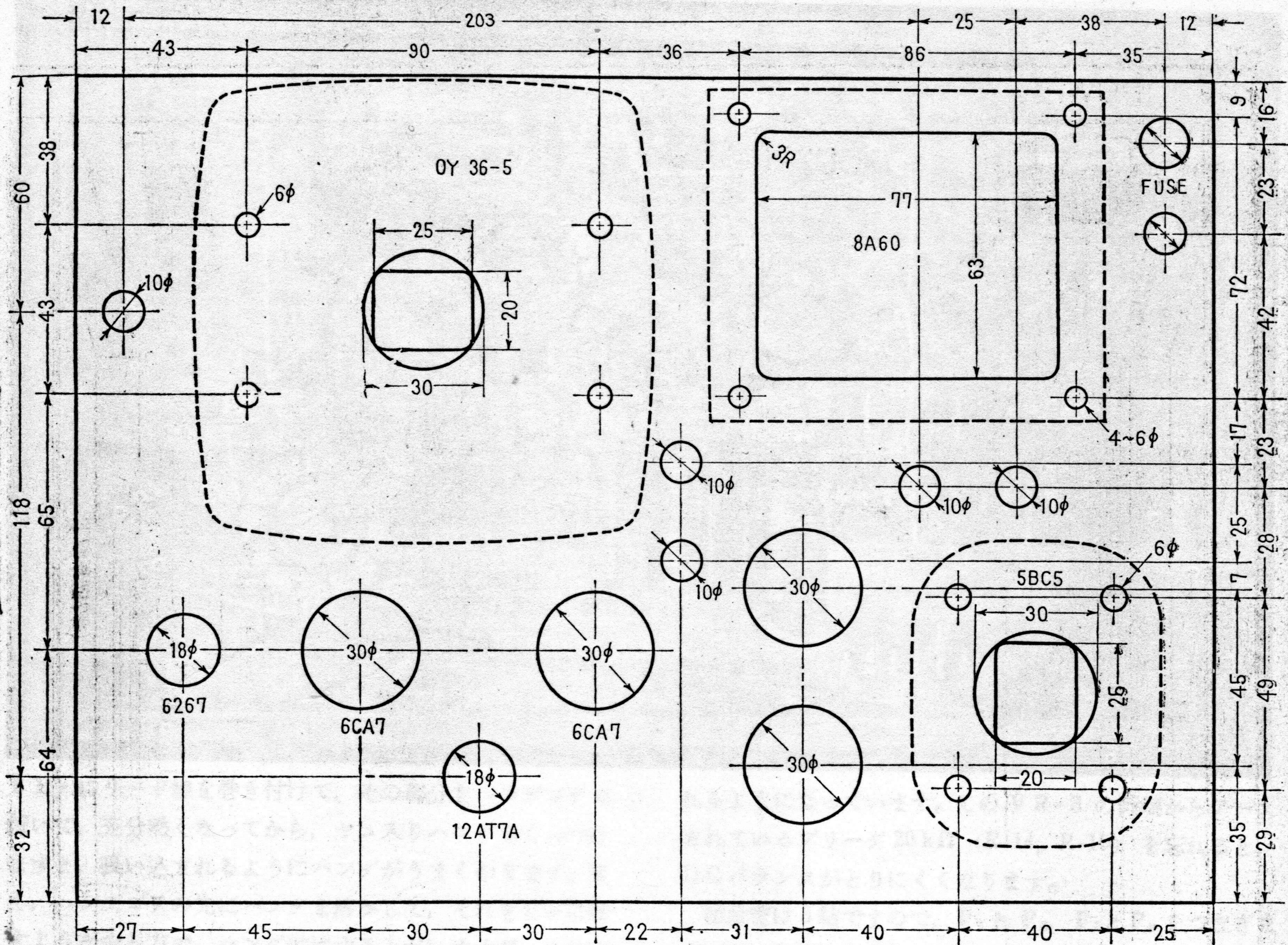
〔第5図〕 シャシ加工図，斜面の部分は使用部品にあわせてあけるため省略，メータは 38 mm φ
