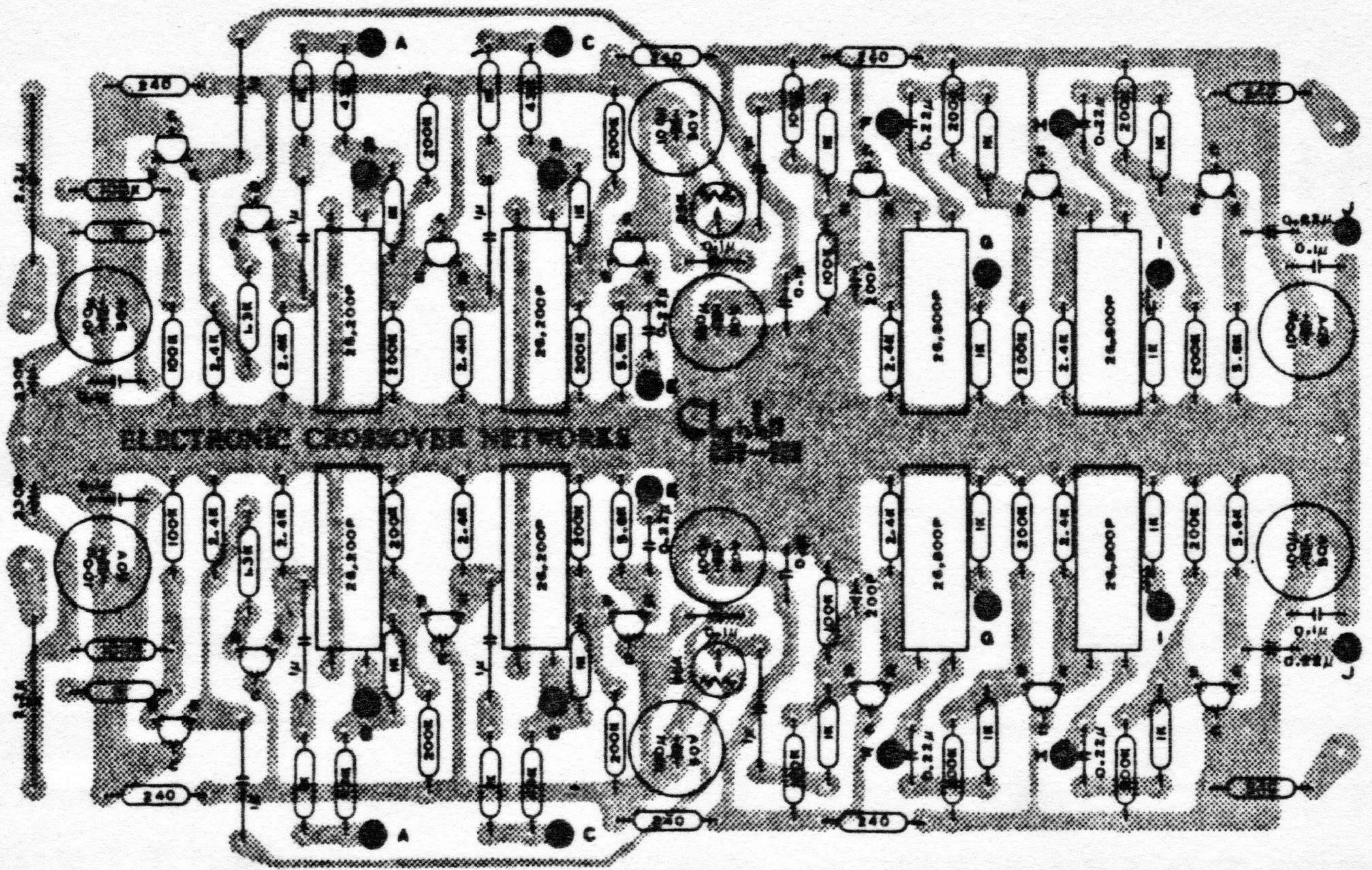
本機のパターン図
