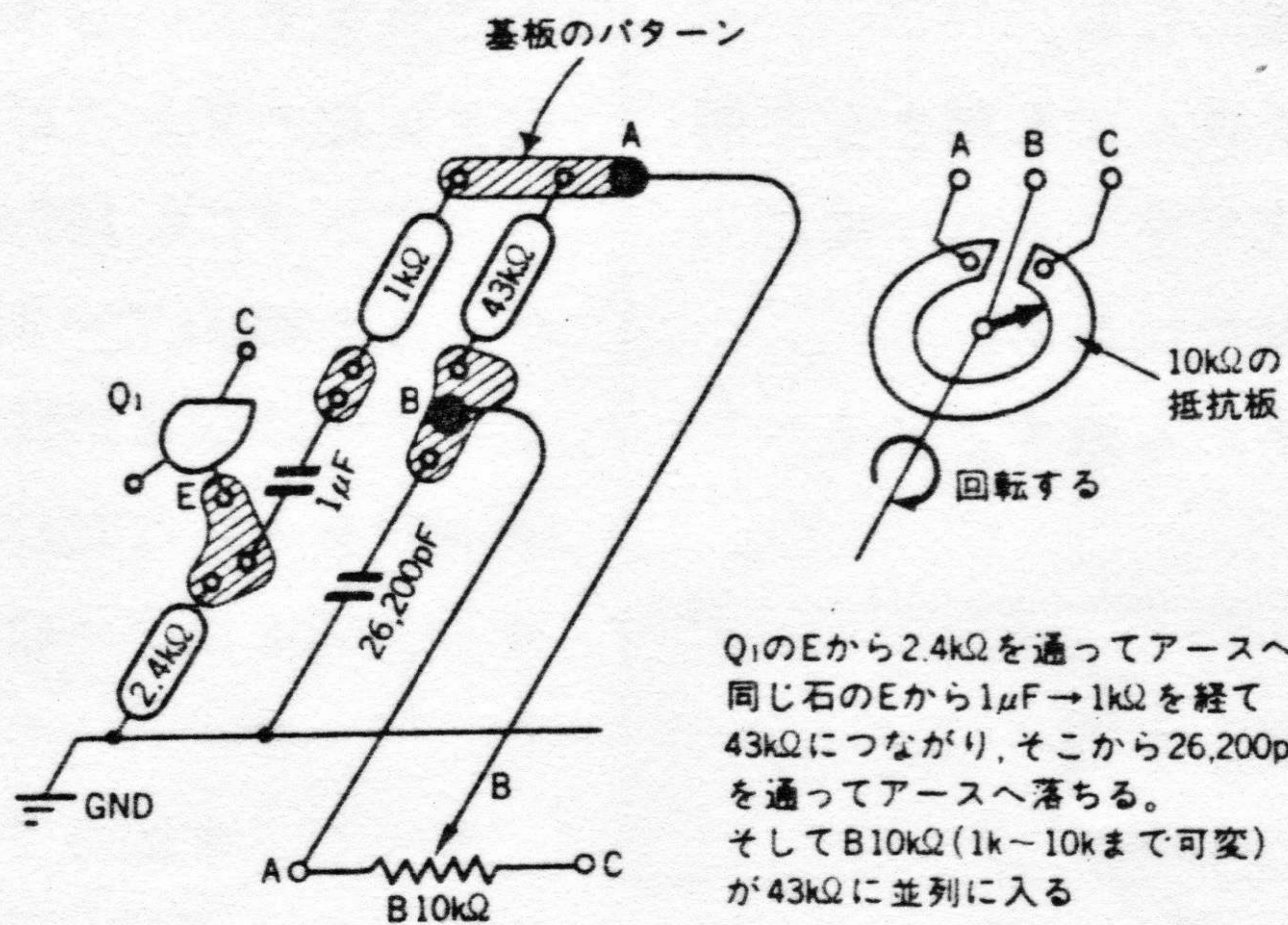
《第20図》実体回路図(Pictorial Schematic)
