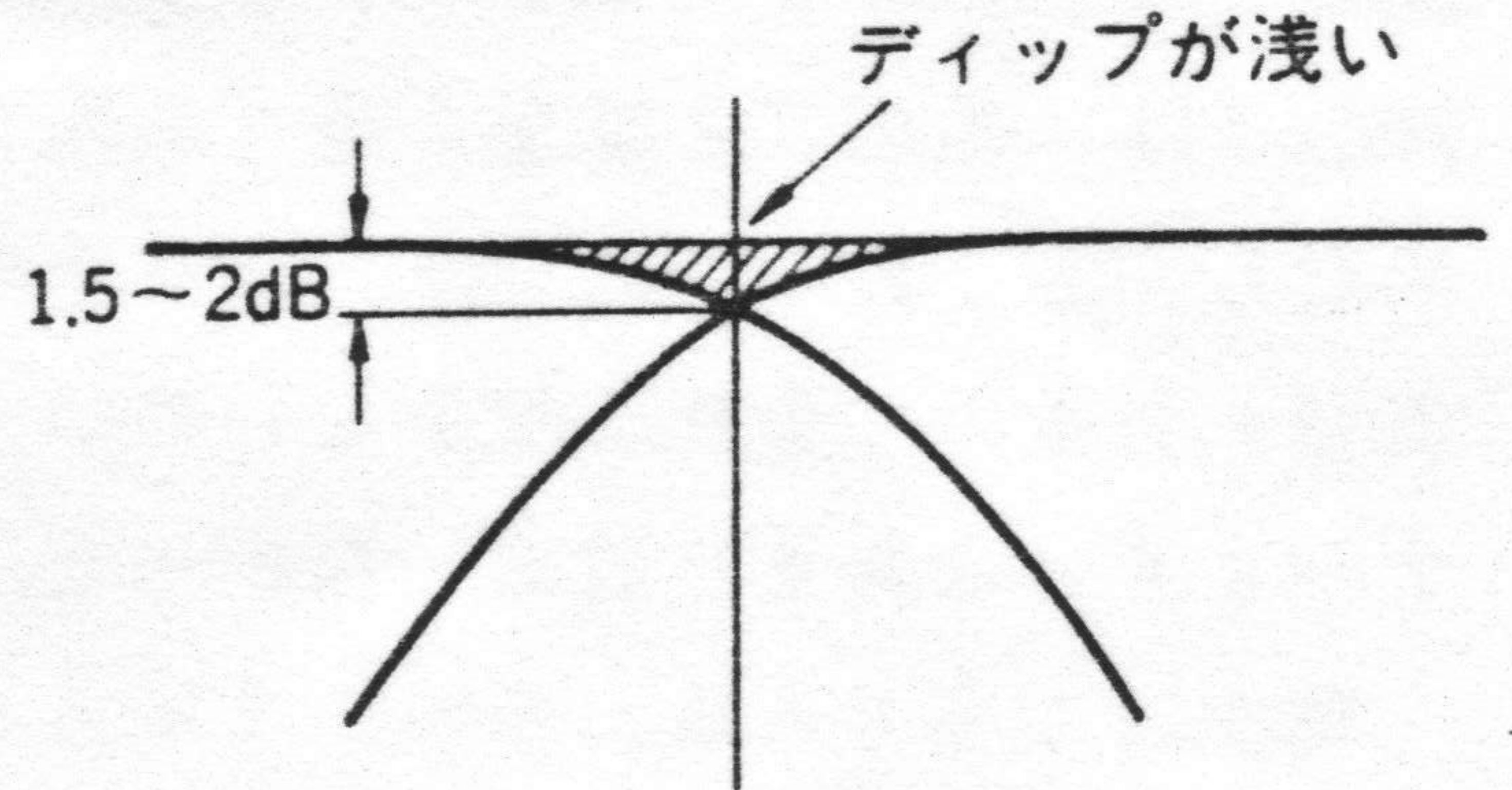
〈第6図〉 マルチスピーカーのクロスオーバー付近のディップ
