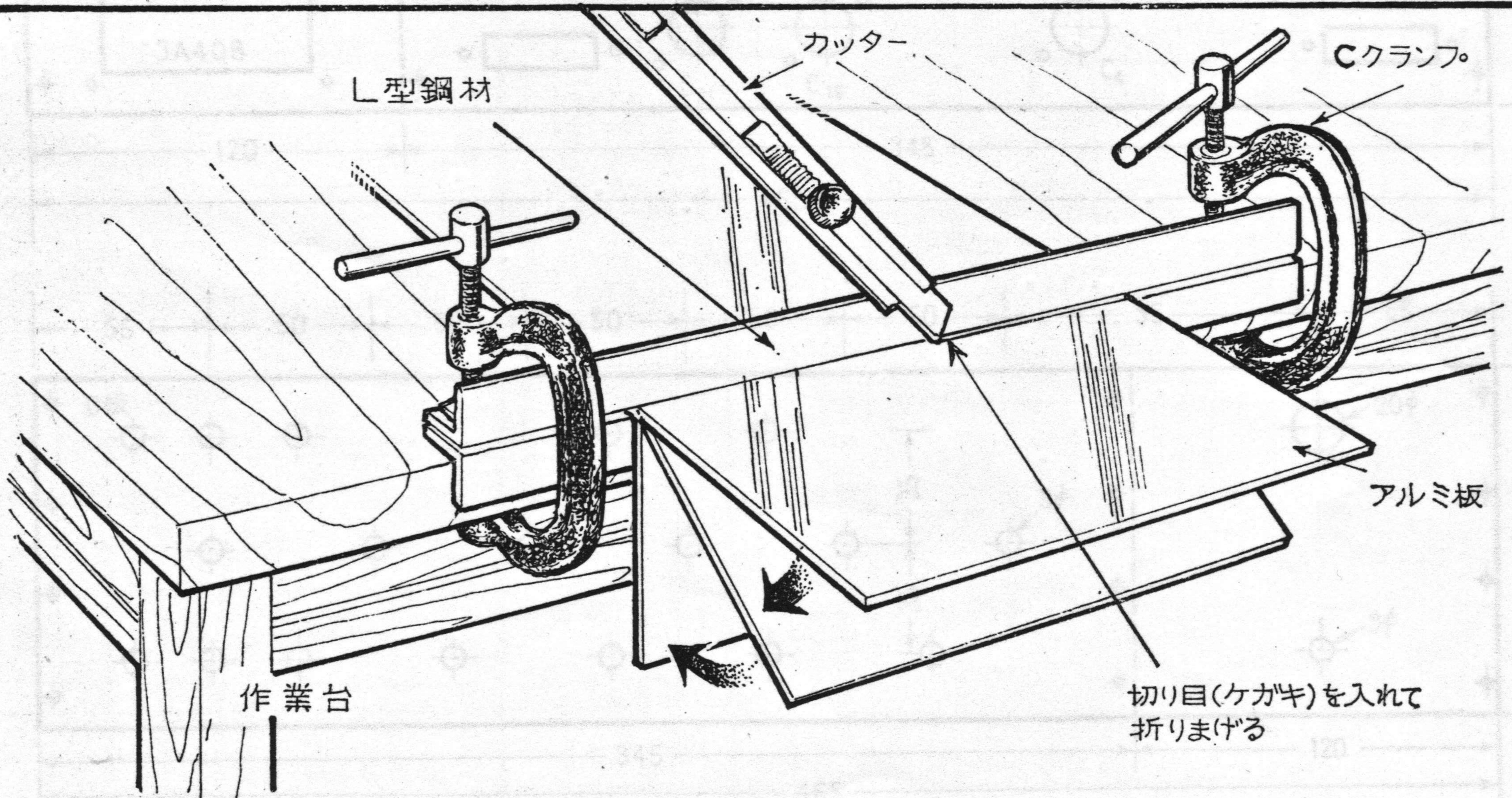
[第9図] アルミ板のまげ方
