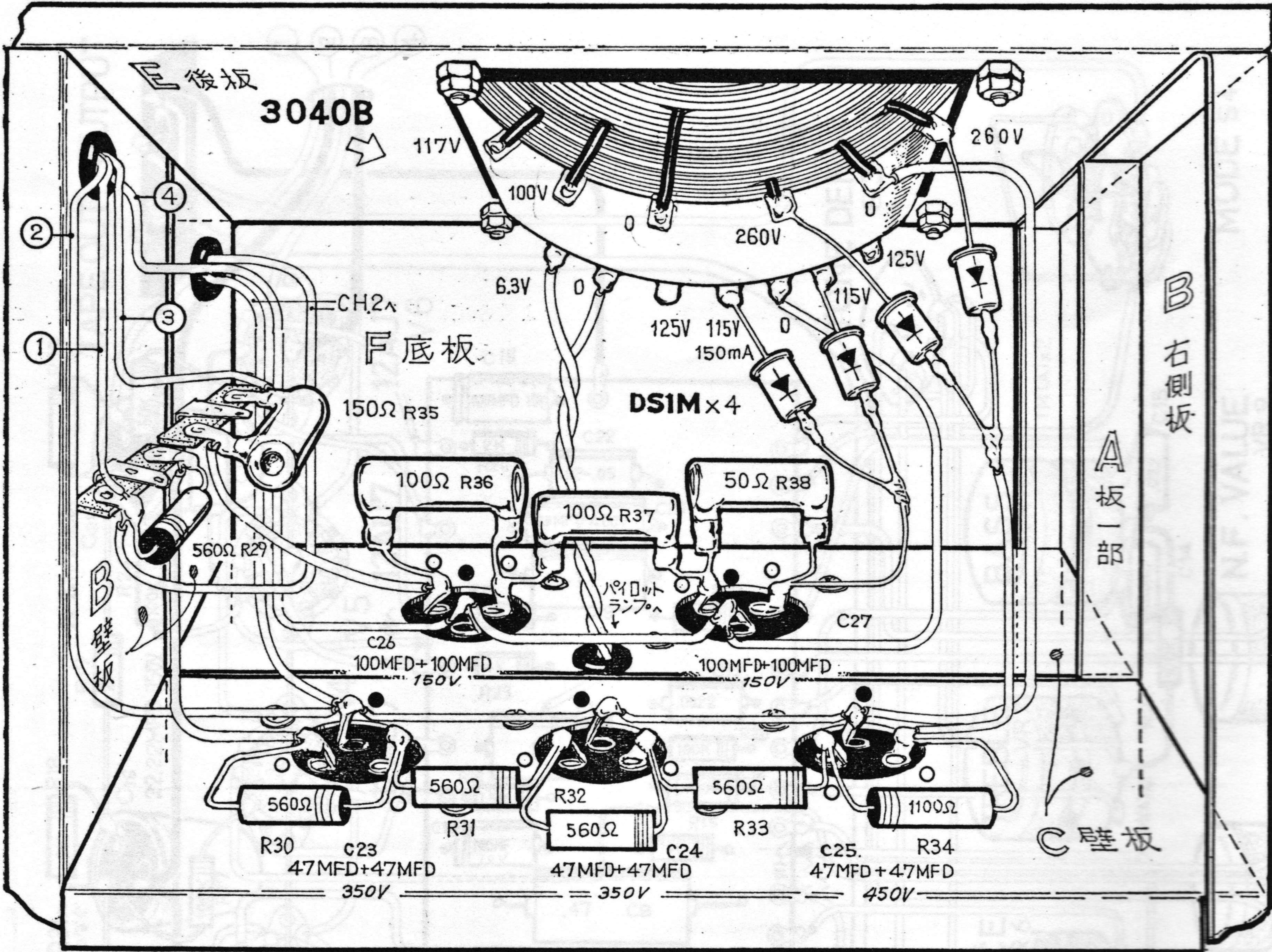
[第14図] 電源部の実体図
