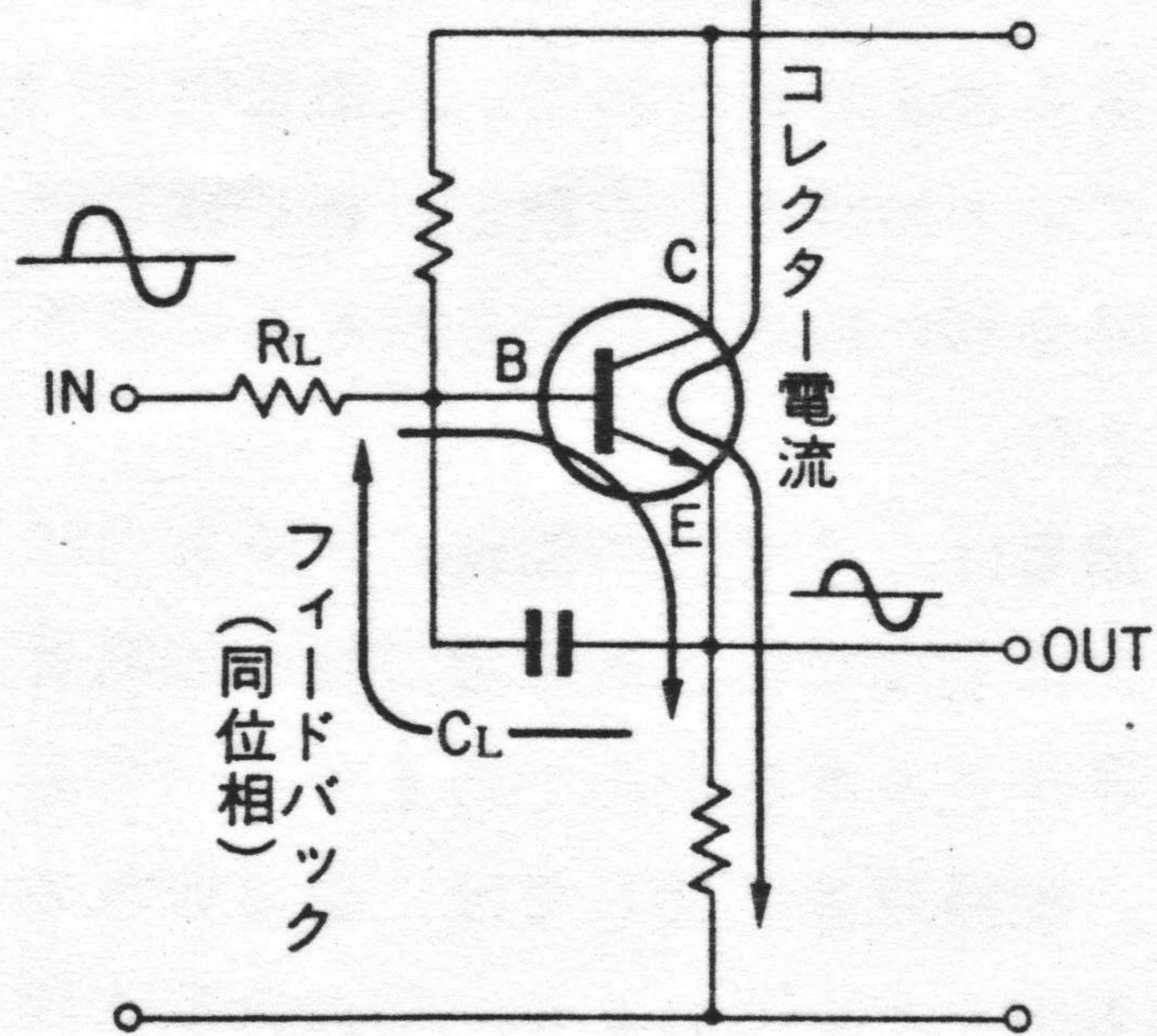
《第4図》トランジスターと真空管のエミッターフォロアー、カソードフォロアーの回路
