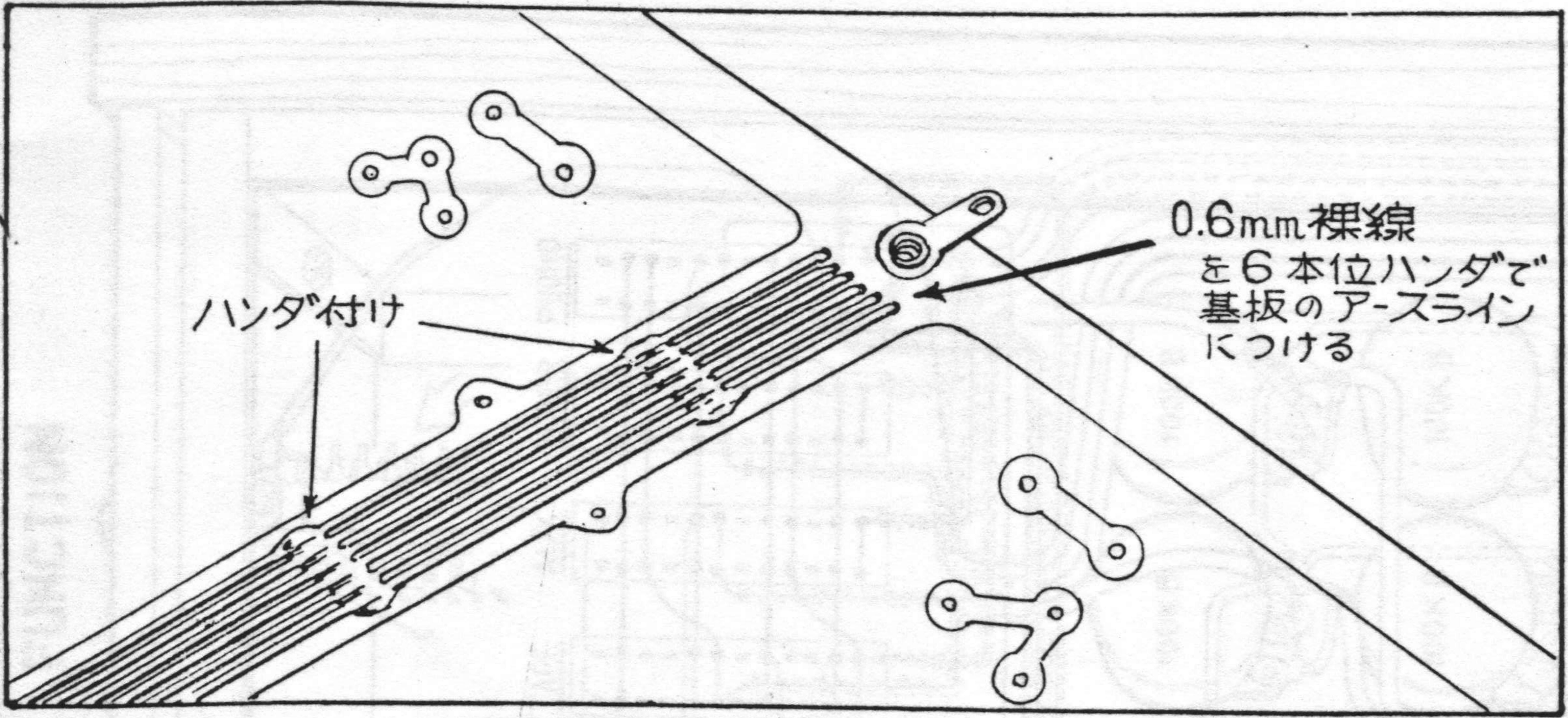
〔第11図〕 プリント基板上的のアースラインのとり方
