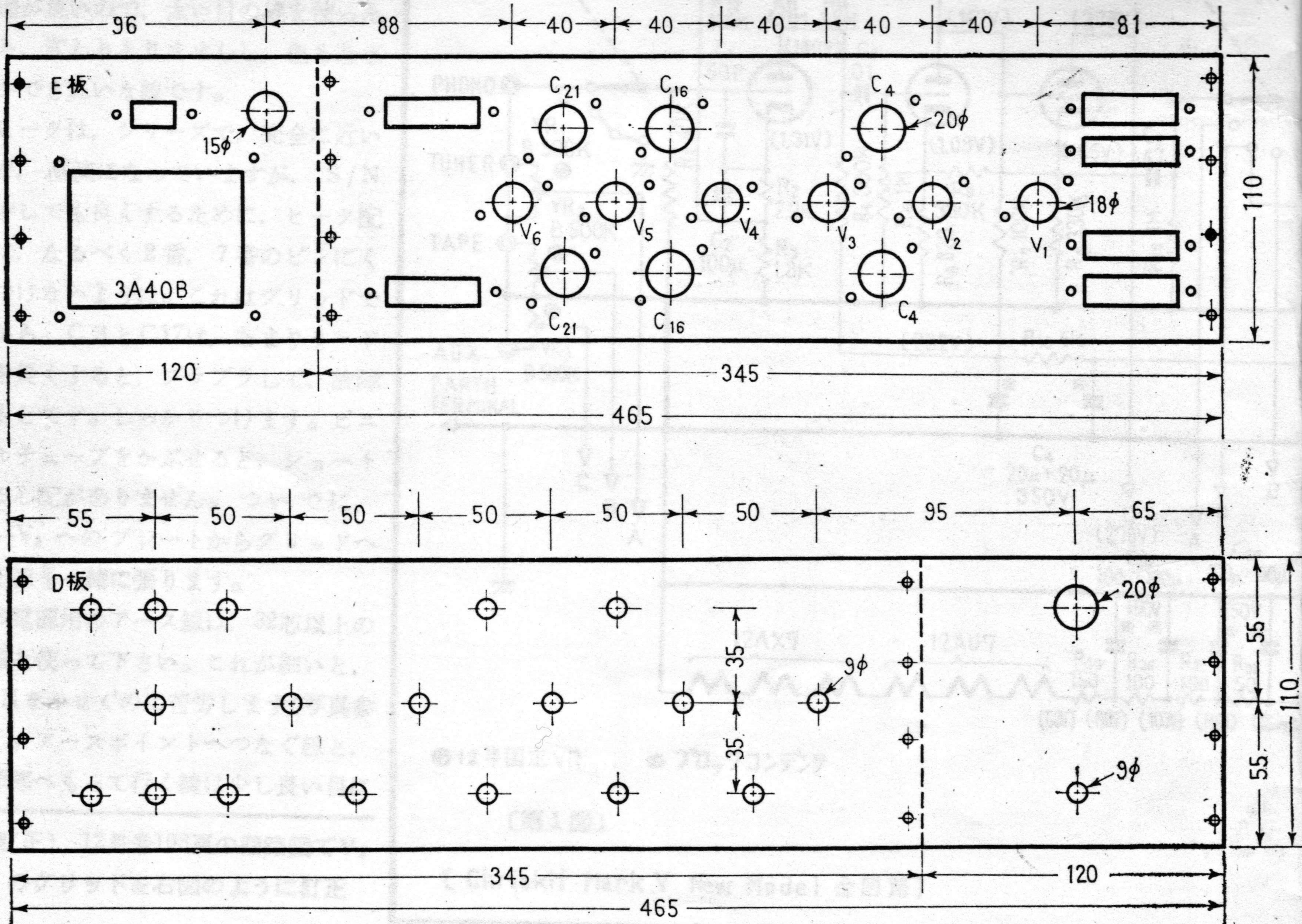
[第10図] b パネル板D~Eの寸法
