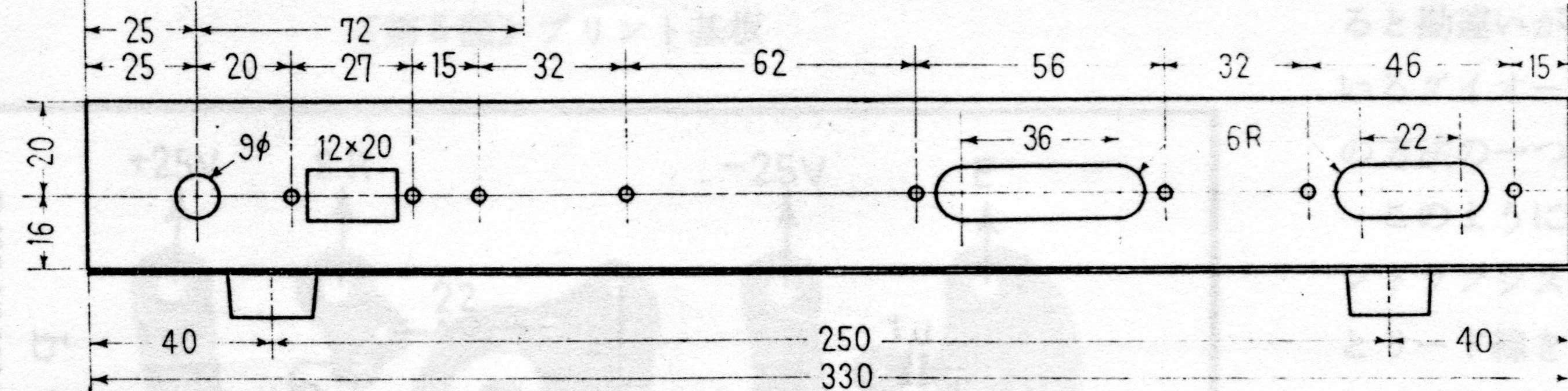
[第2図] シ ャ シ 寸 法 図
