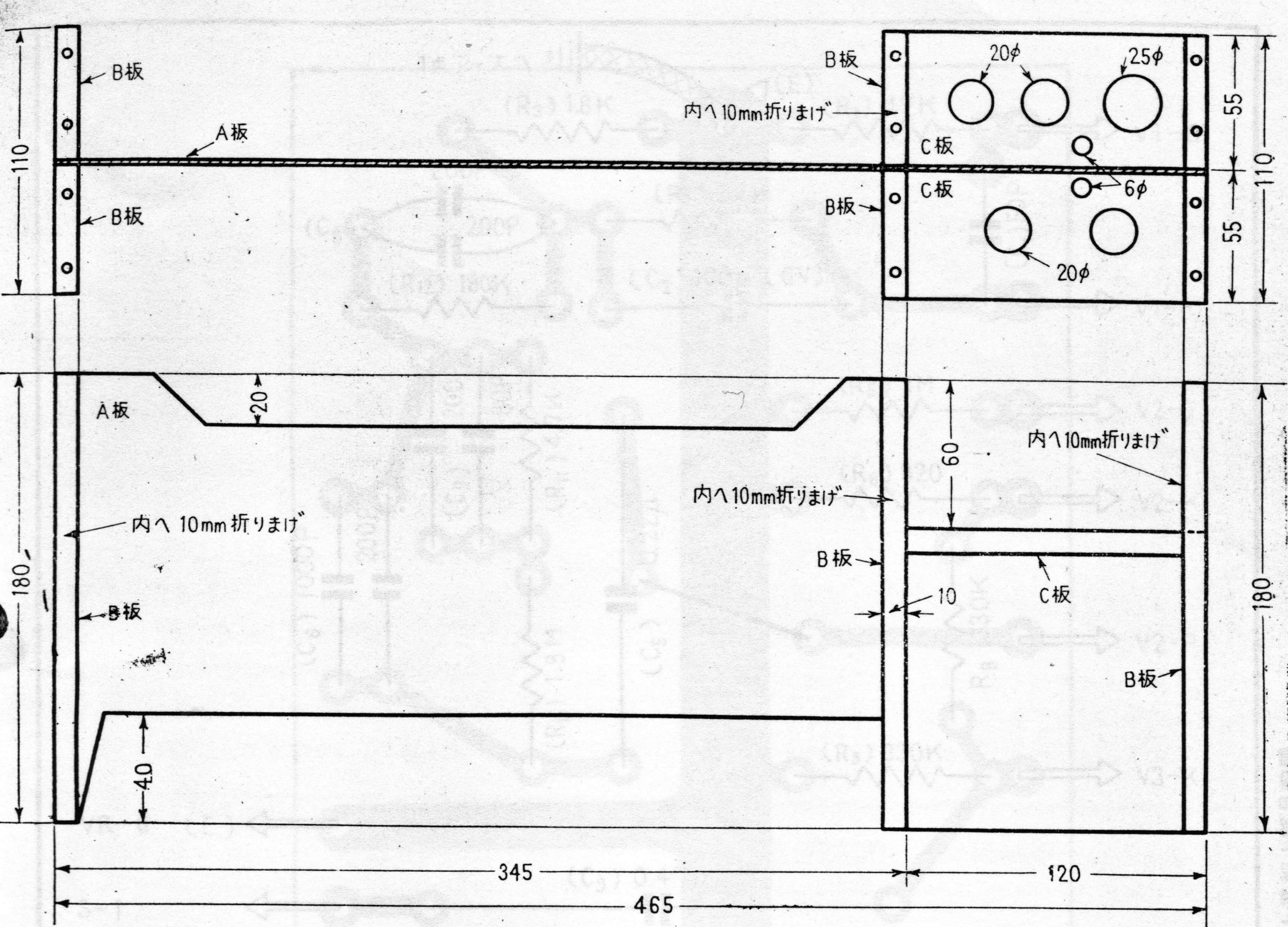
〔第10図〕 a シャシA~Cの寸法
