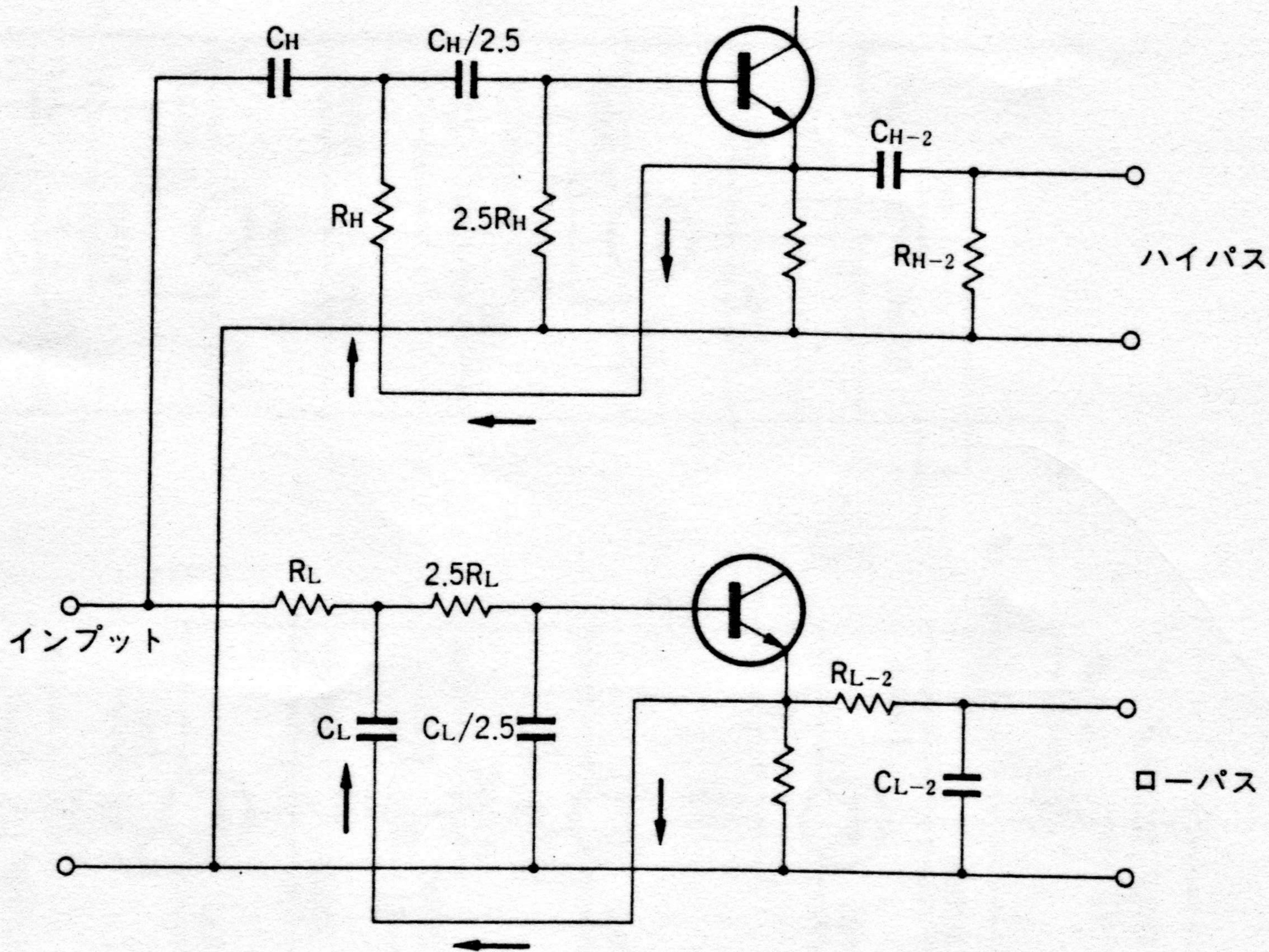
〈第7図〉 -18\text{dB/oct} 山根式チャンネルデバイダーの基本回路
