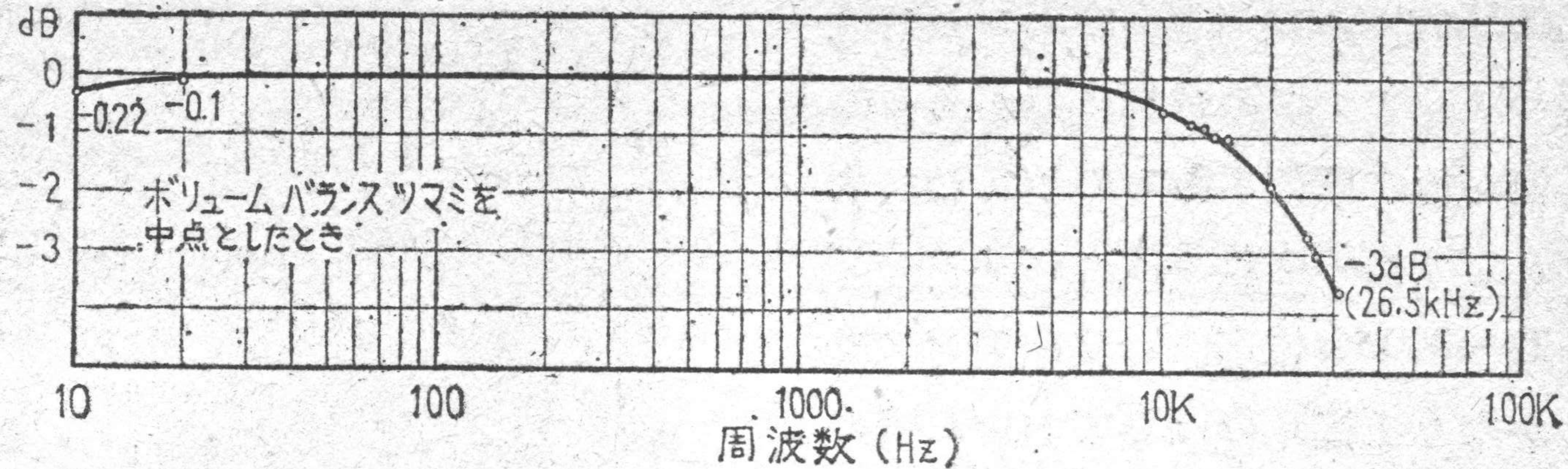
〔第5図〕 周波数特性
