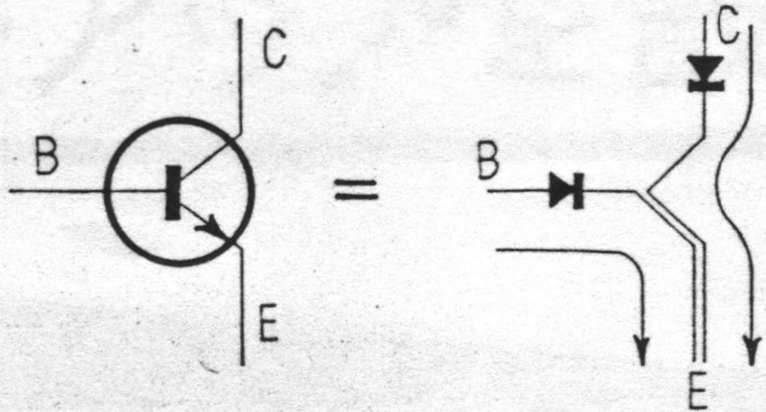
(a) NPNの場合
