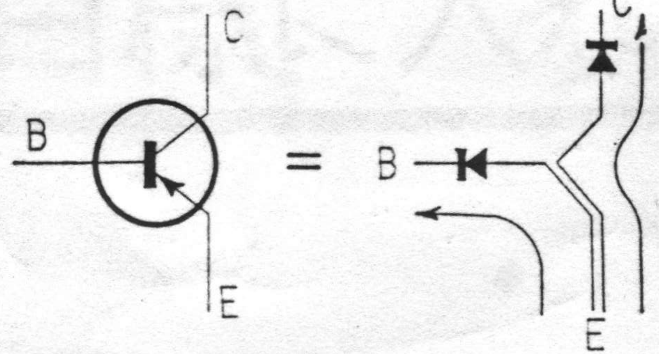
(b) PNPの場合
