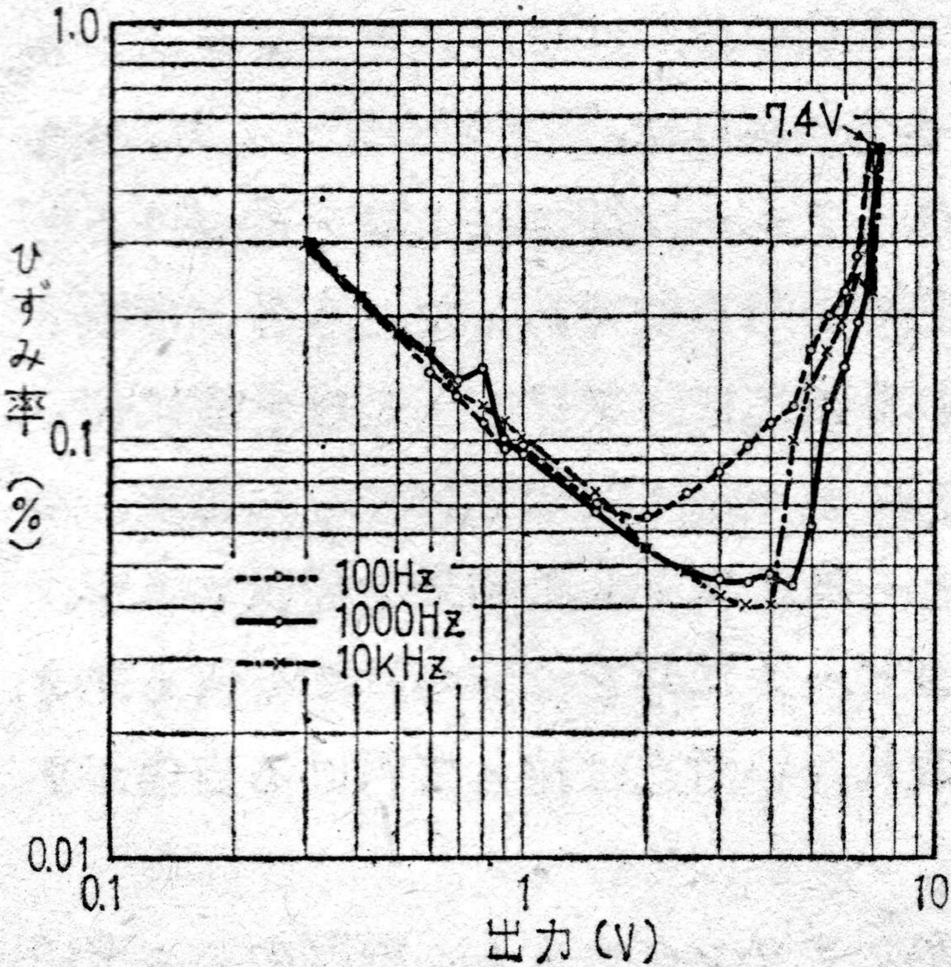
[第8図] イコライザの歪率特性
