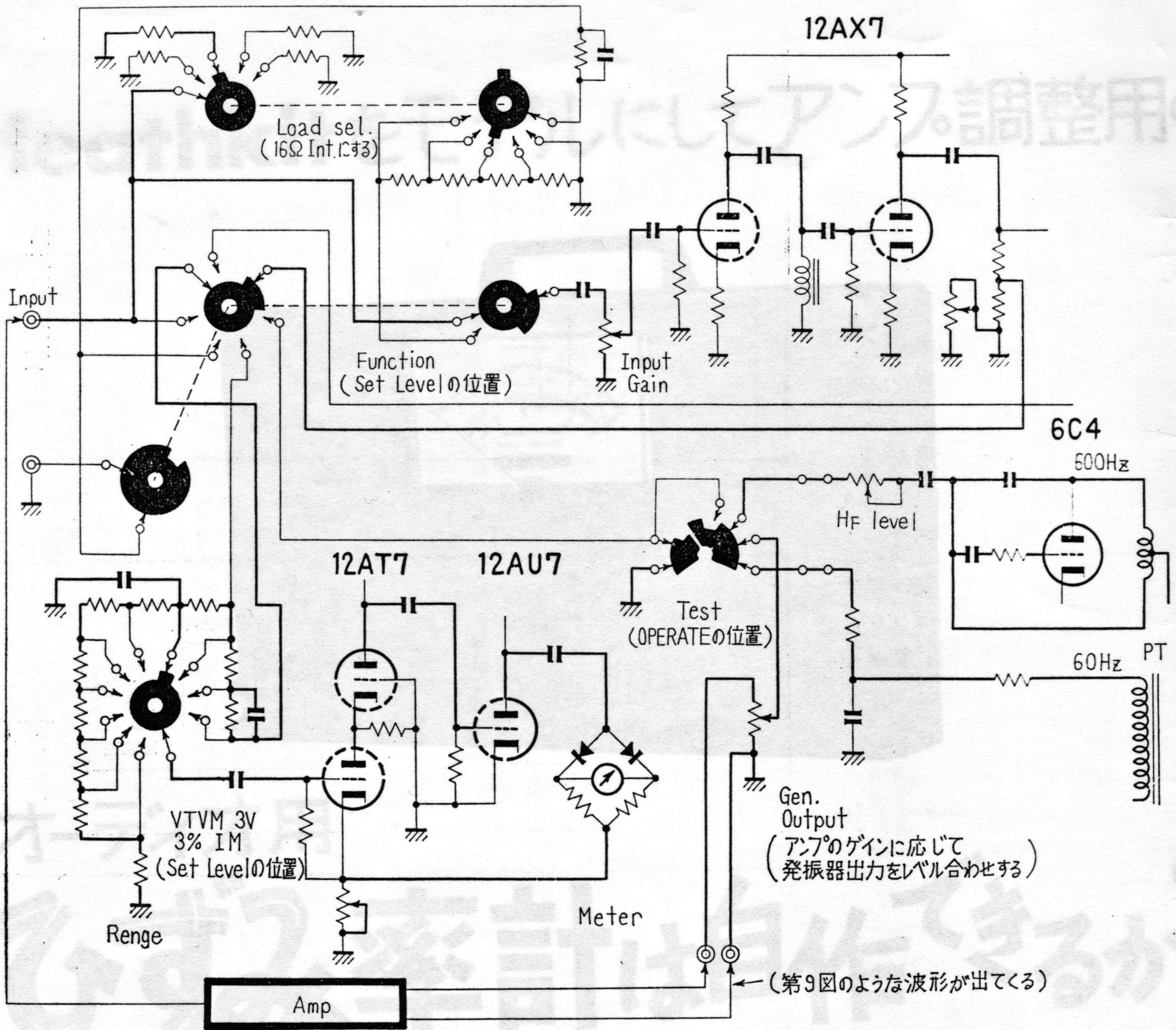
[第8図] アンプ測定回路
