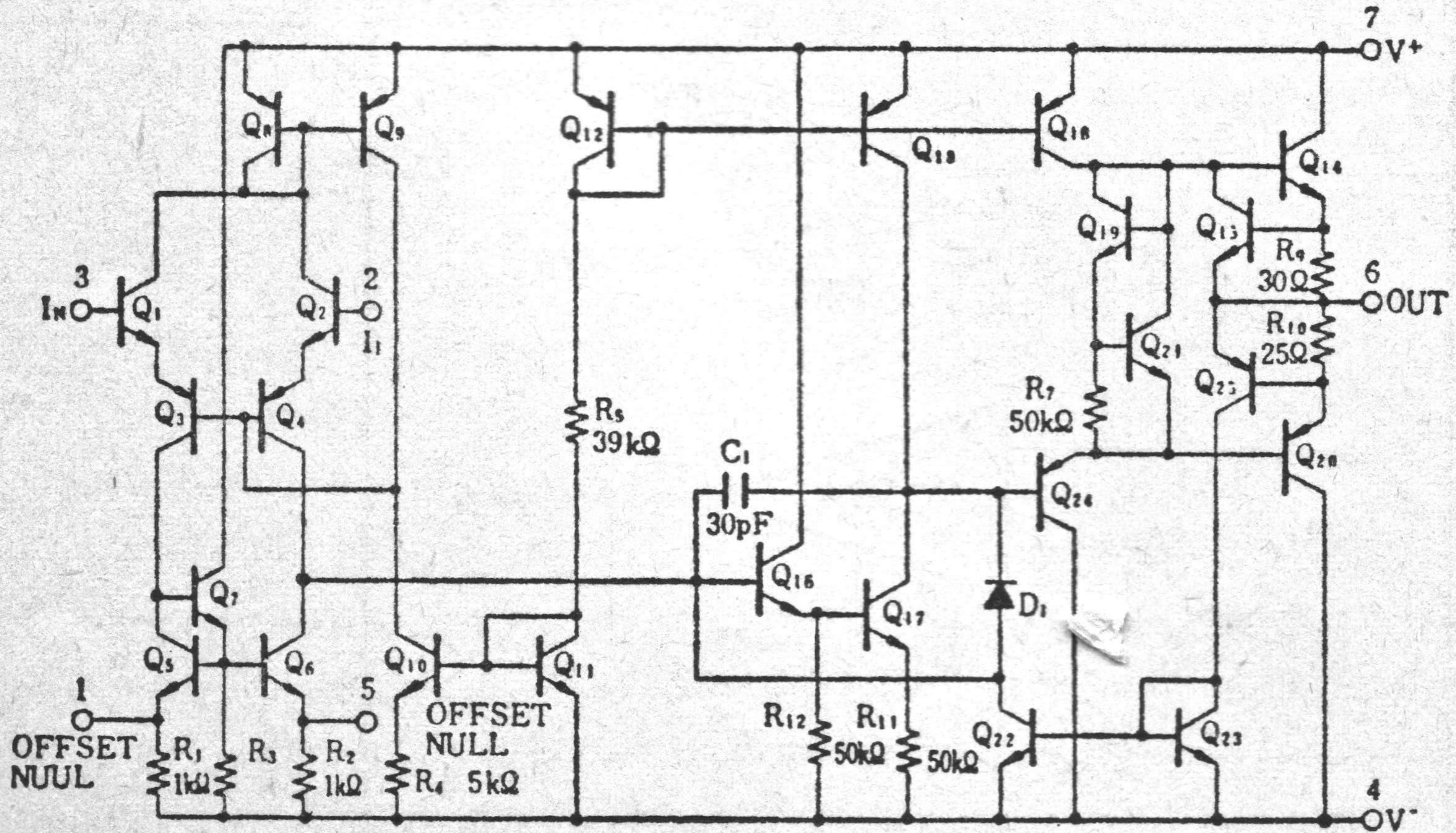
[第1図] \mu\text{PC151A} の等価回路
