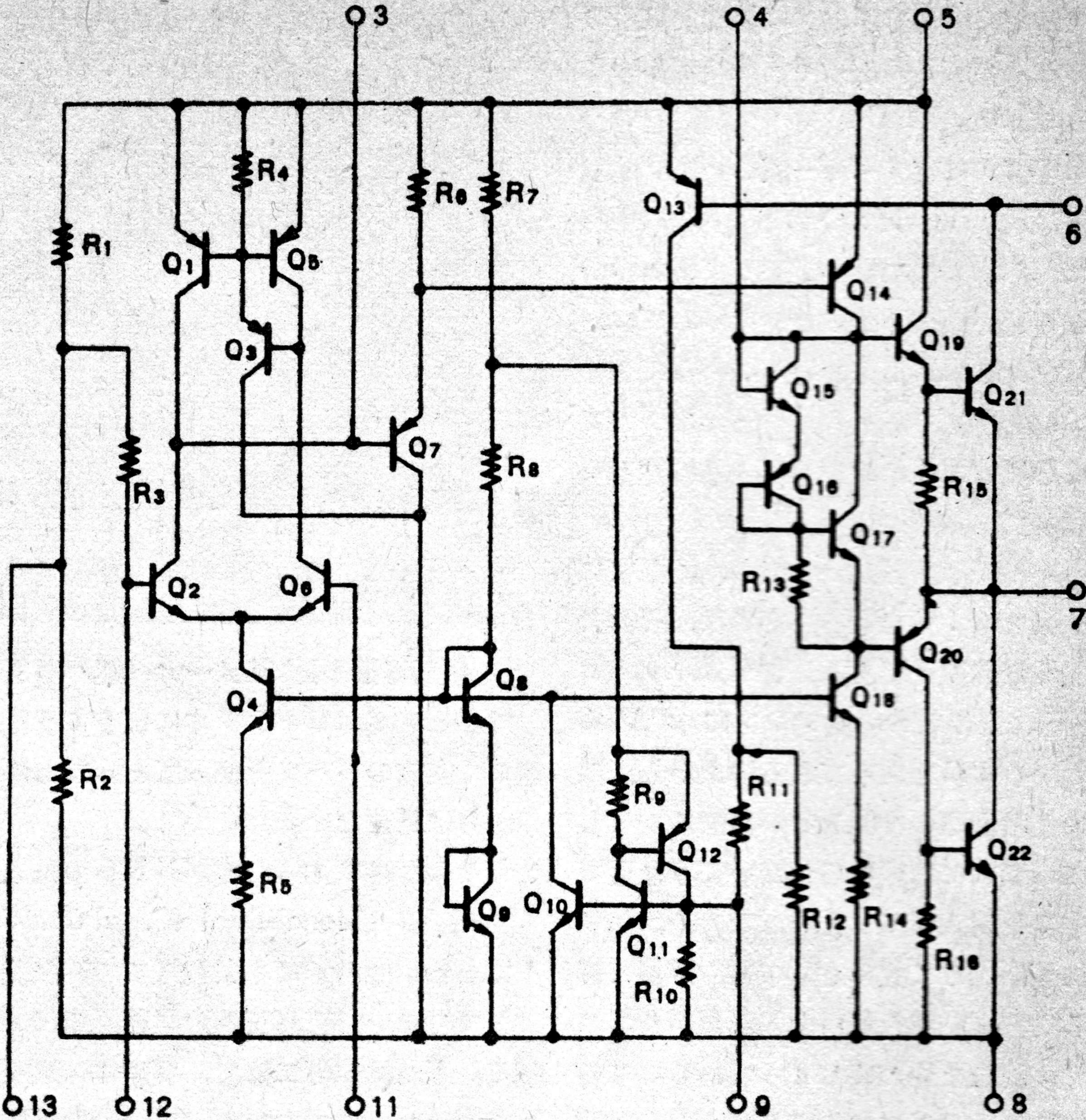
[第1図] ICの内部回路
