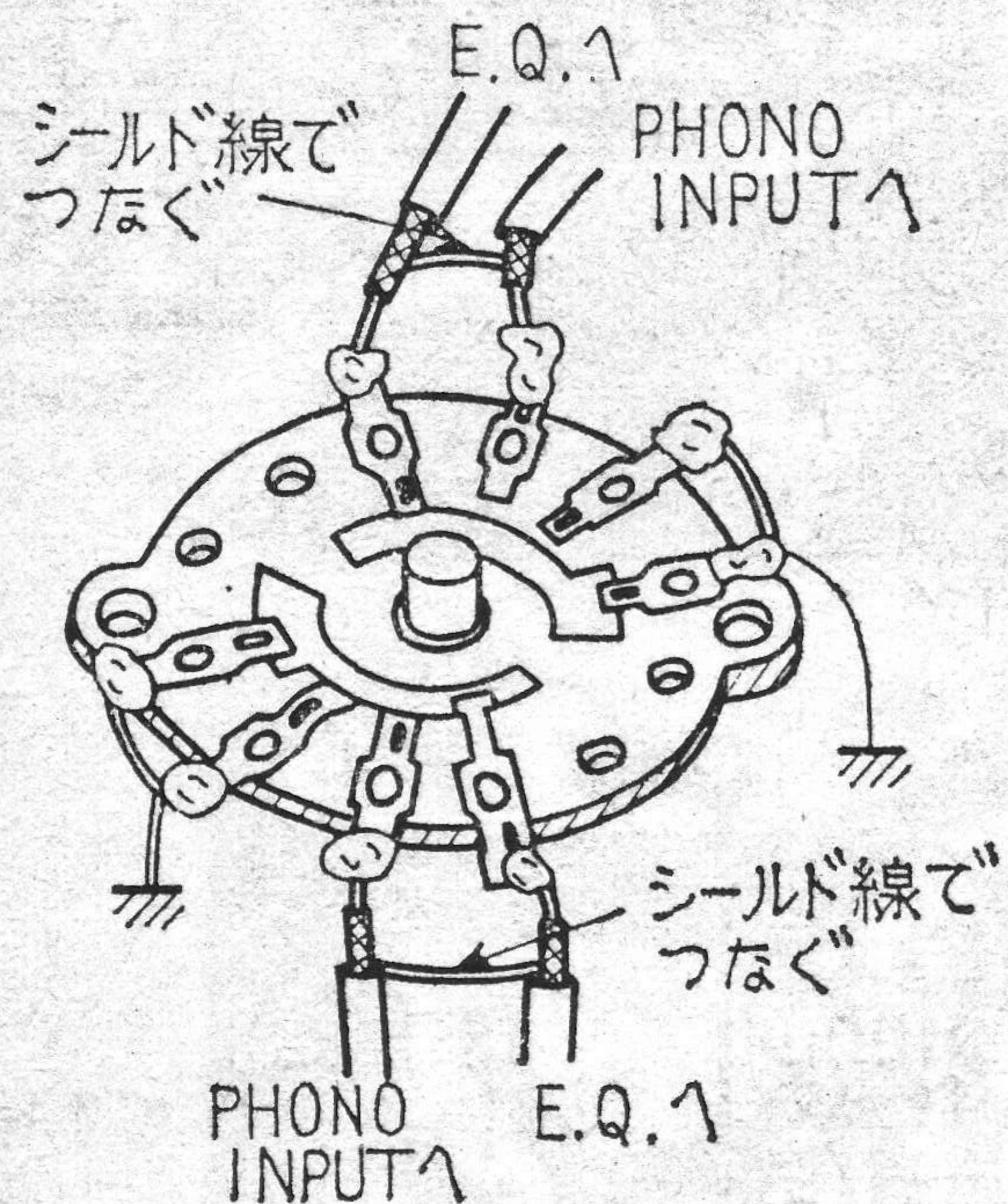
(a) 実体配線図
