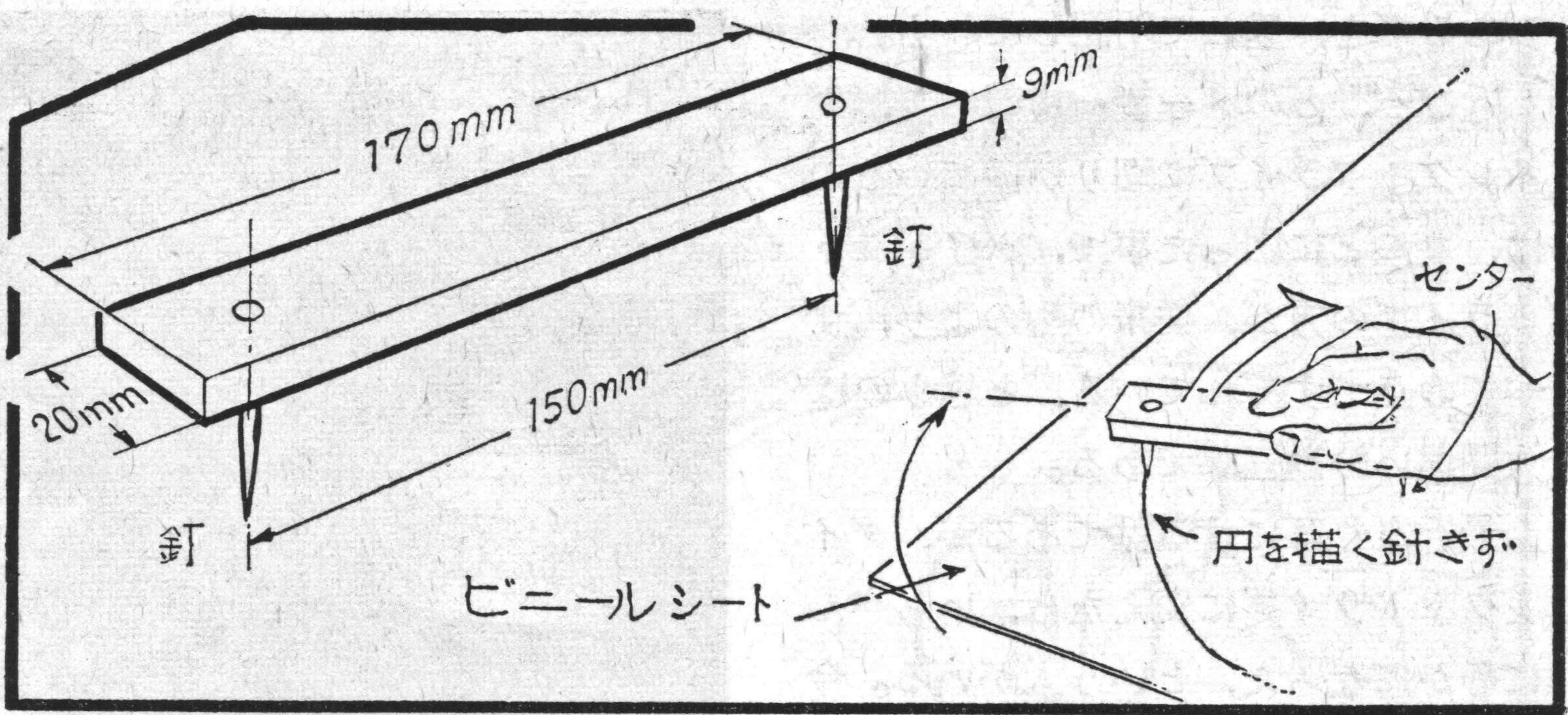
〔第1図〕 ビニールシートを丸形に切り抜く
