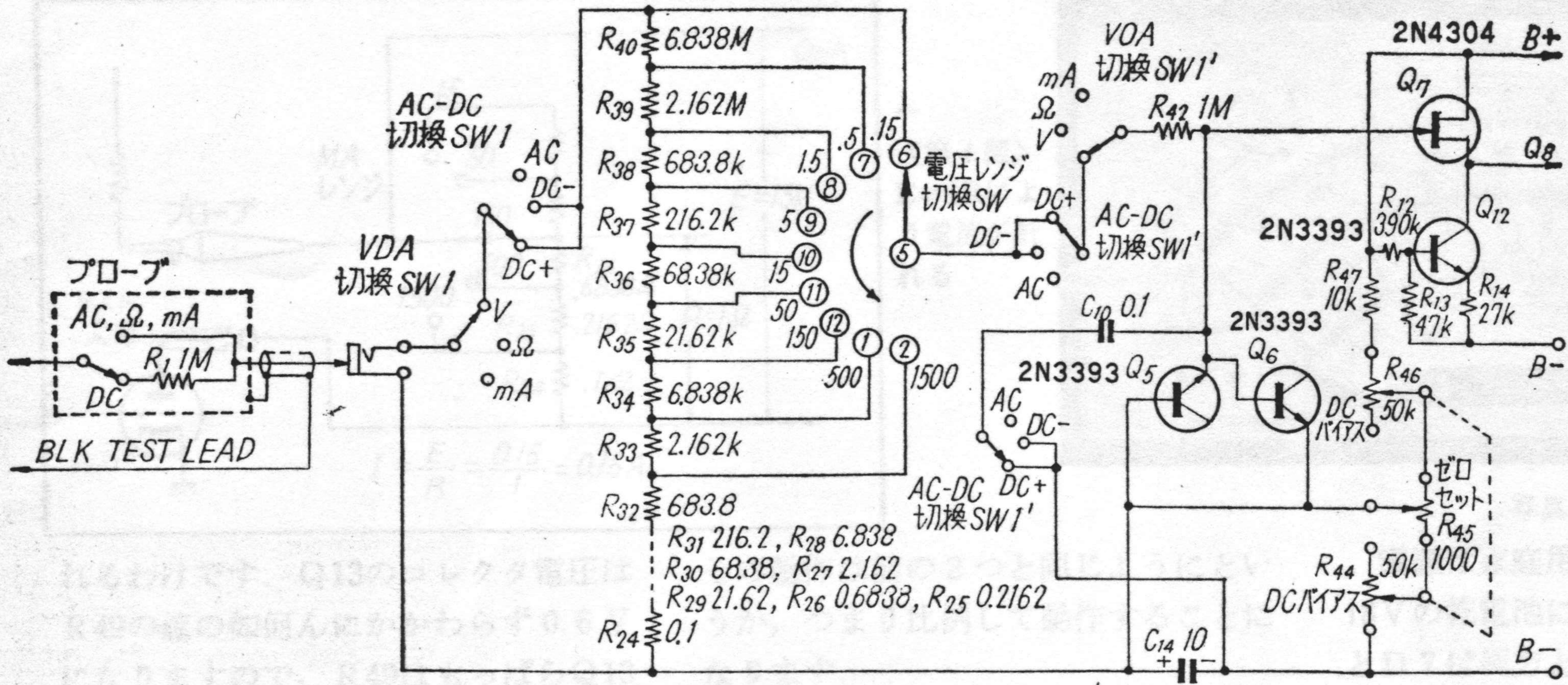
←〈第2図〉 全回路図から DC 電圧測定部をとり だして考える
