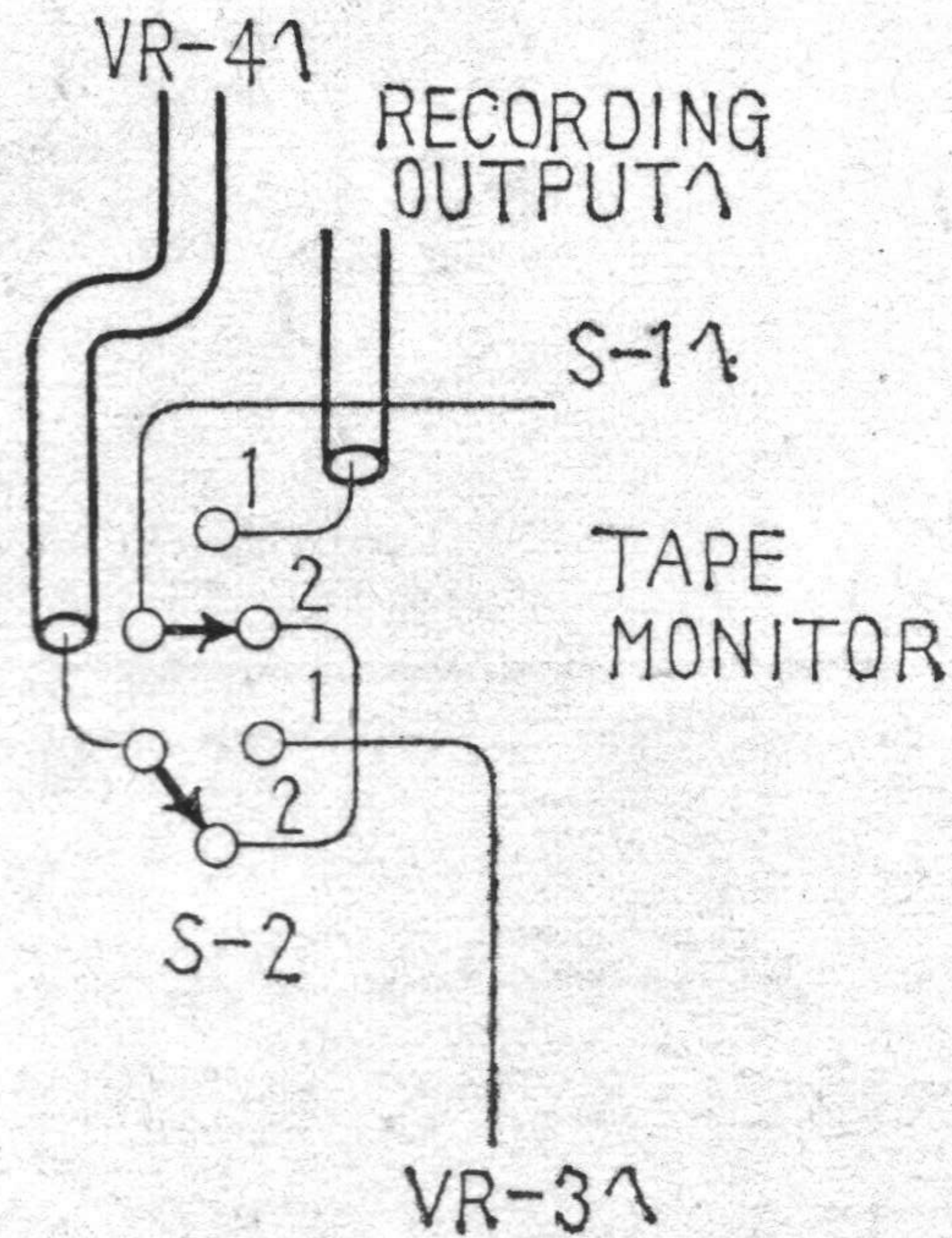
(b) 実体回路図
