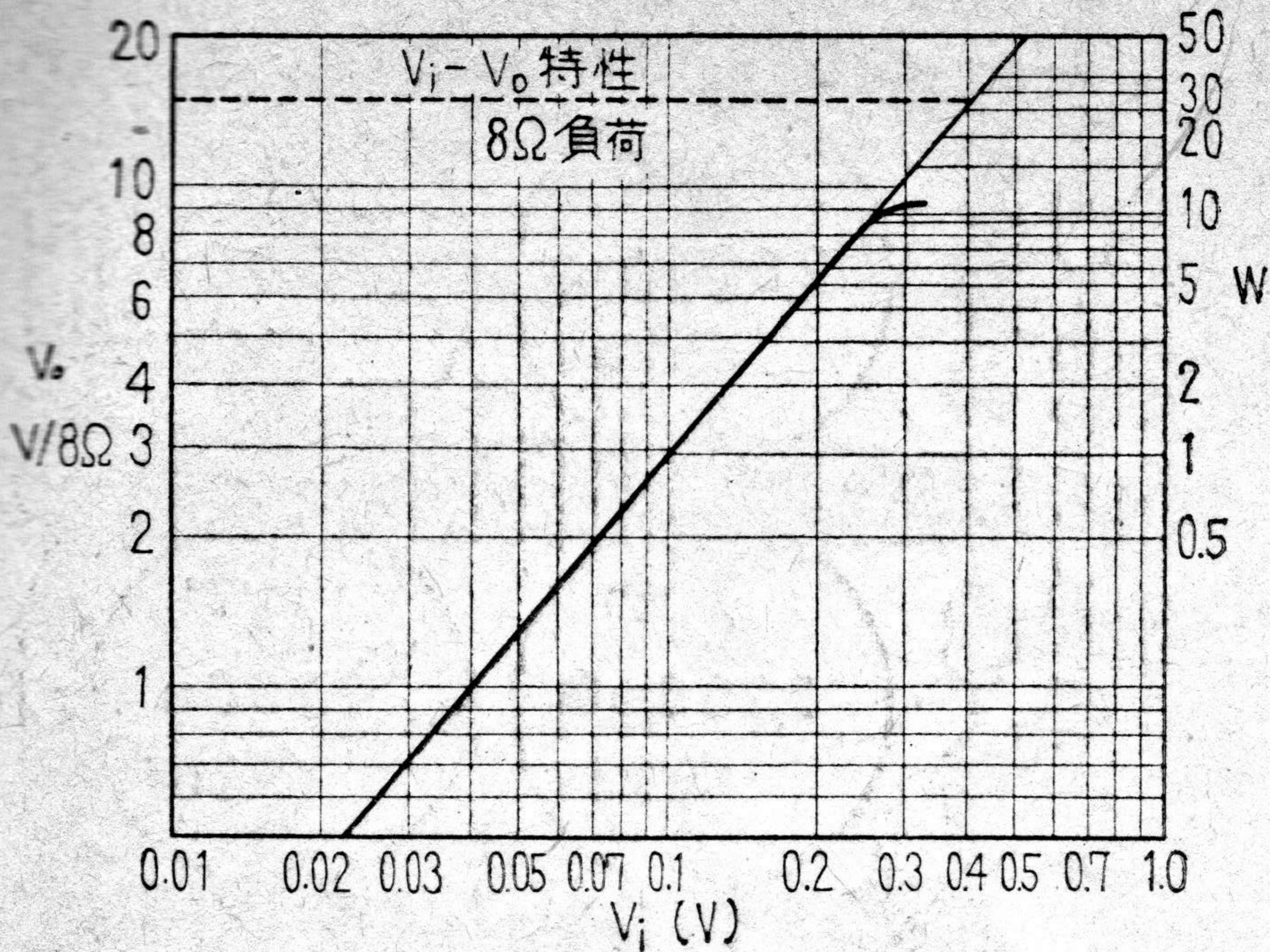
〔第4図〕 入出力特性
