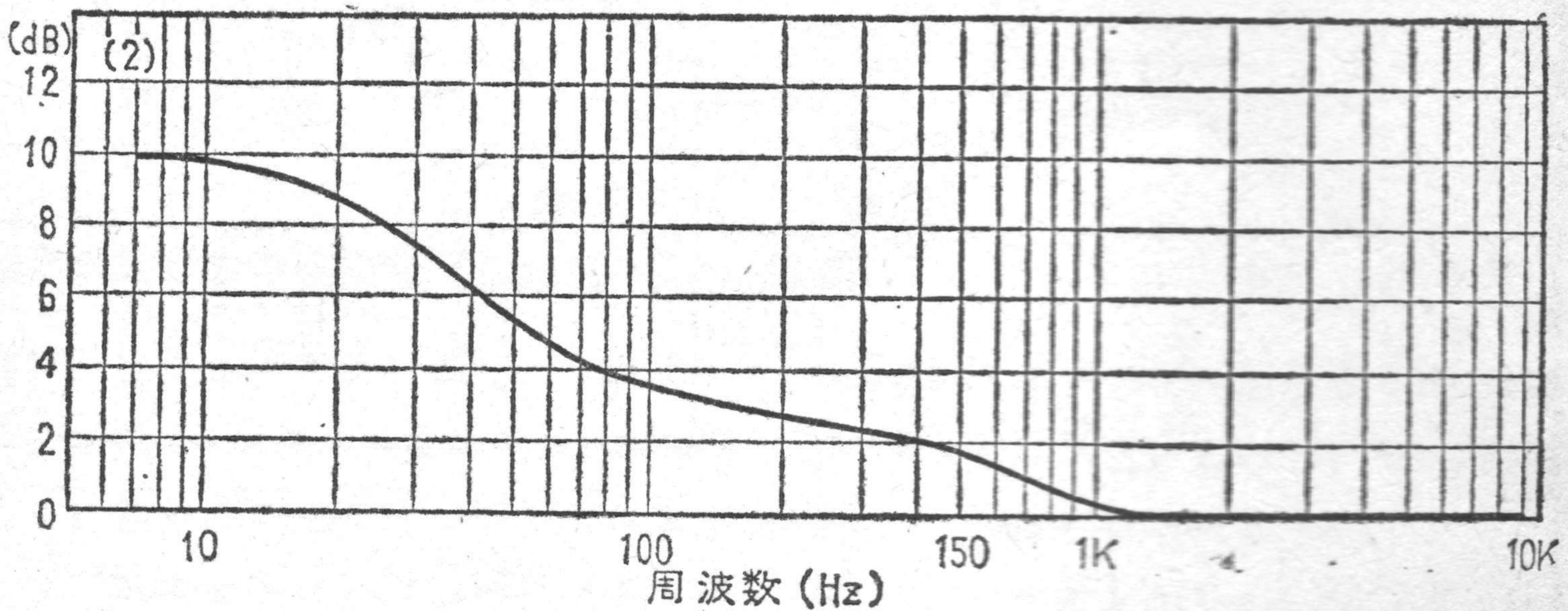
〔第4図〕 トーンコントロールの特性
