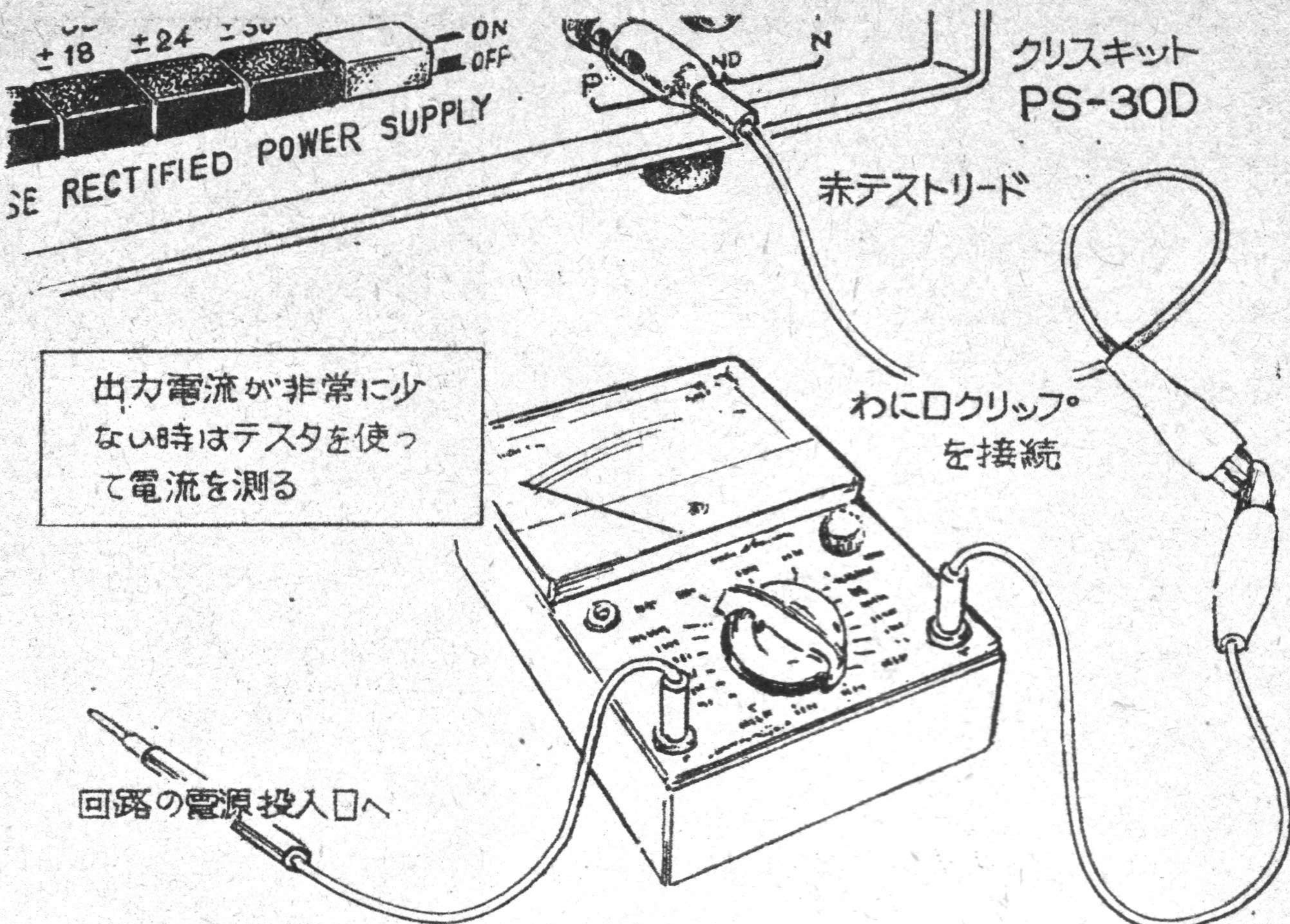
〔第4図〕 ミリアンペアを測るとき
