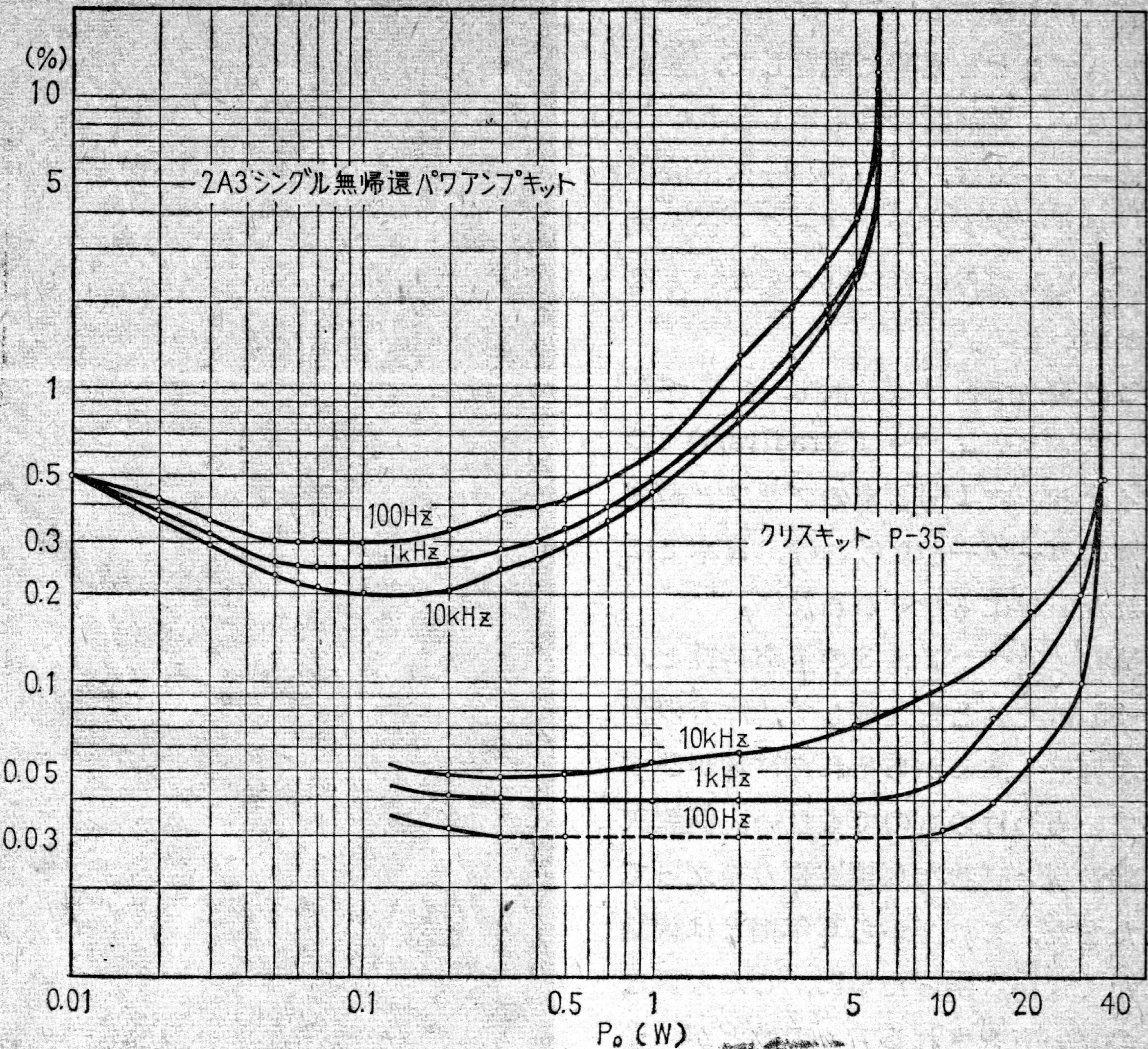
〔第47図〕 出力対歪率特性
