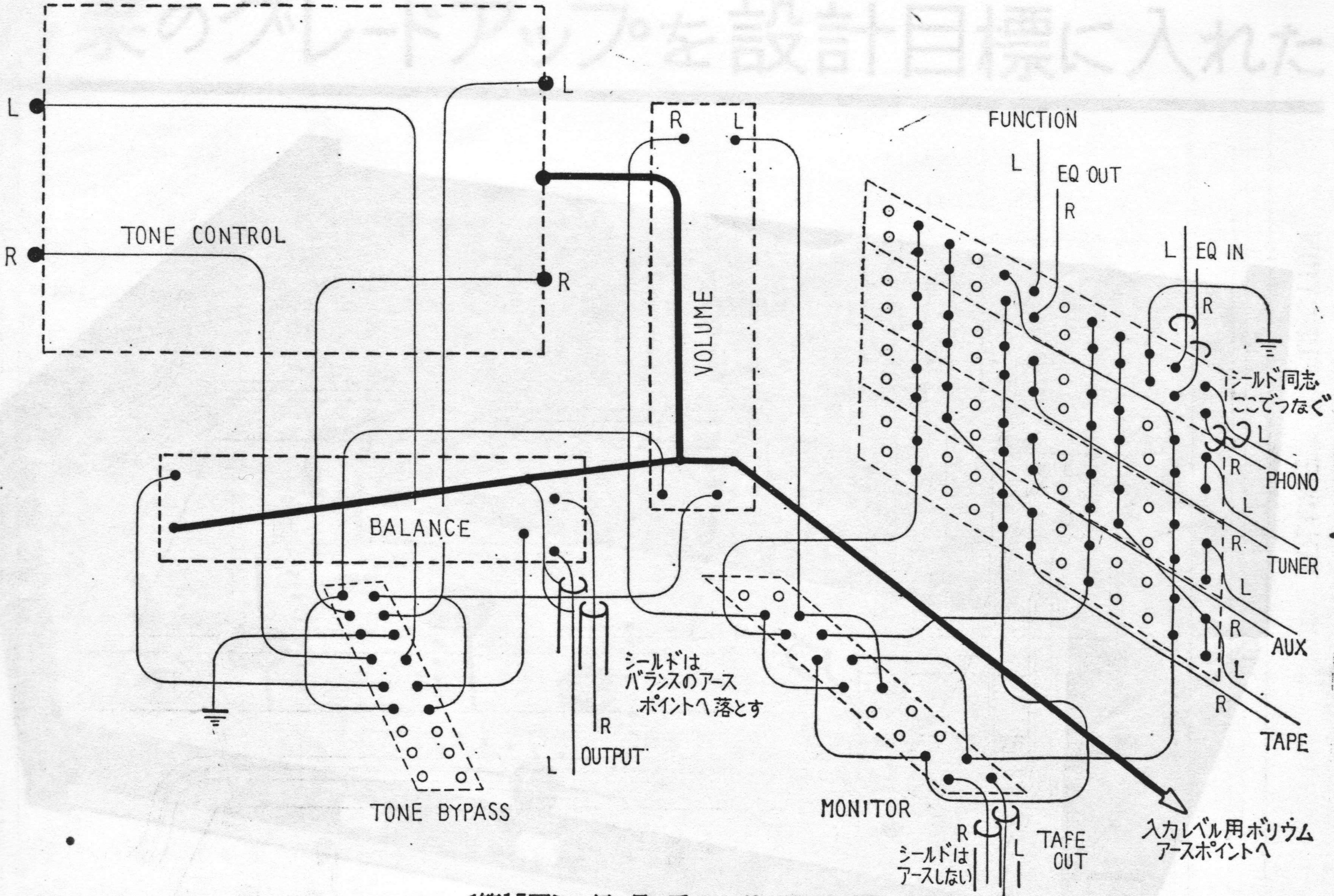
[第15図] 信号系立体回路図
