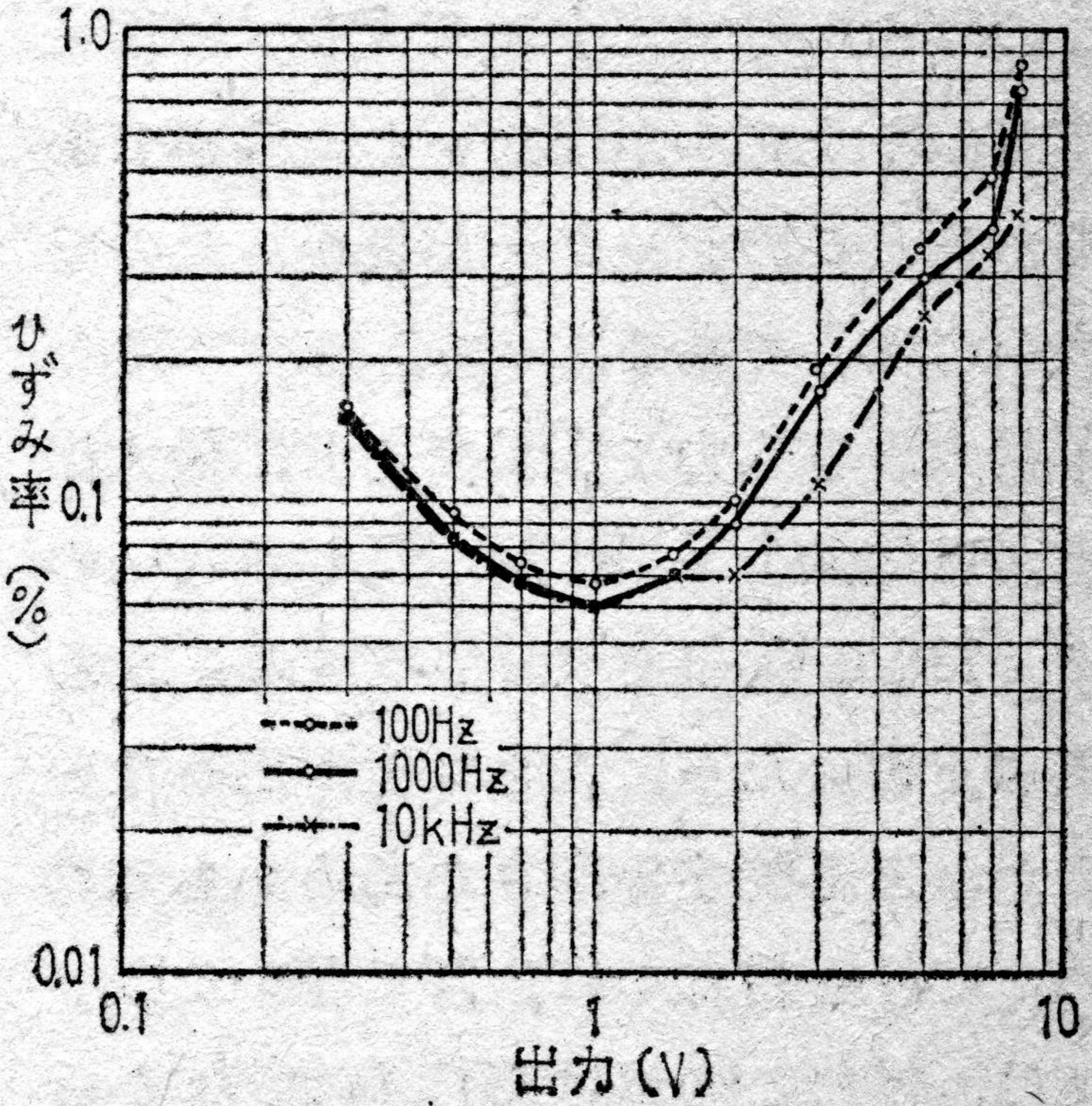
[第9図] フラットアンプの歪率特性
