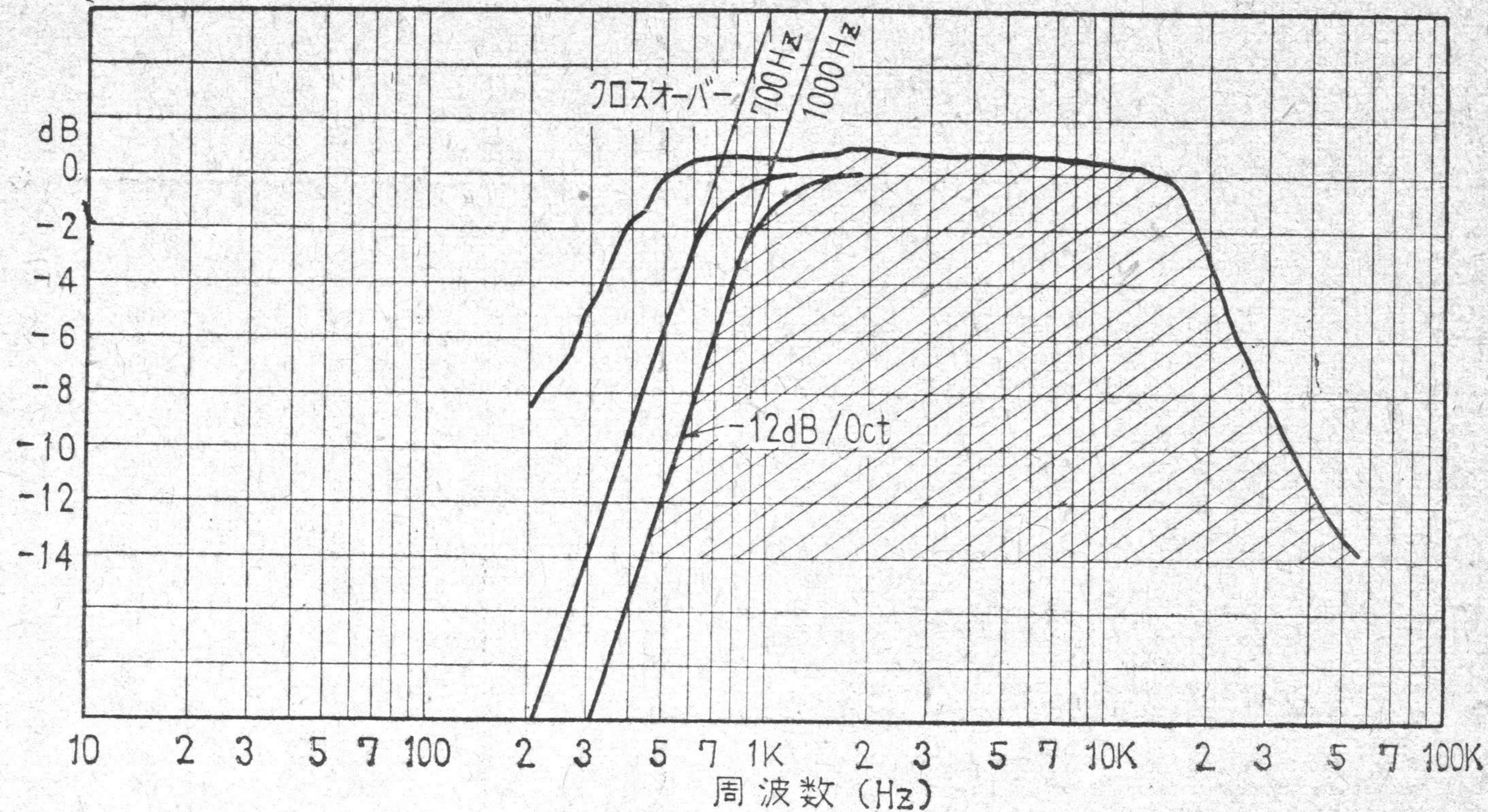
〔第48図〕 クロスオーバー周波数特性
