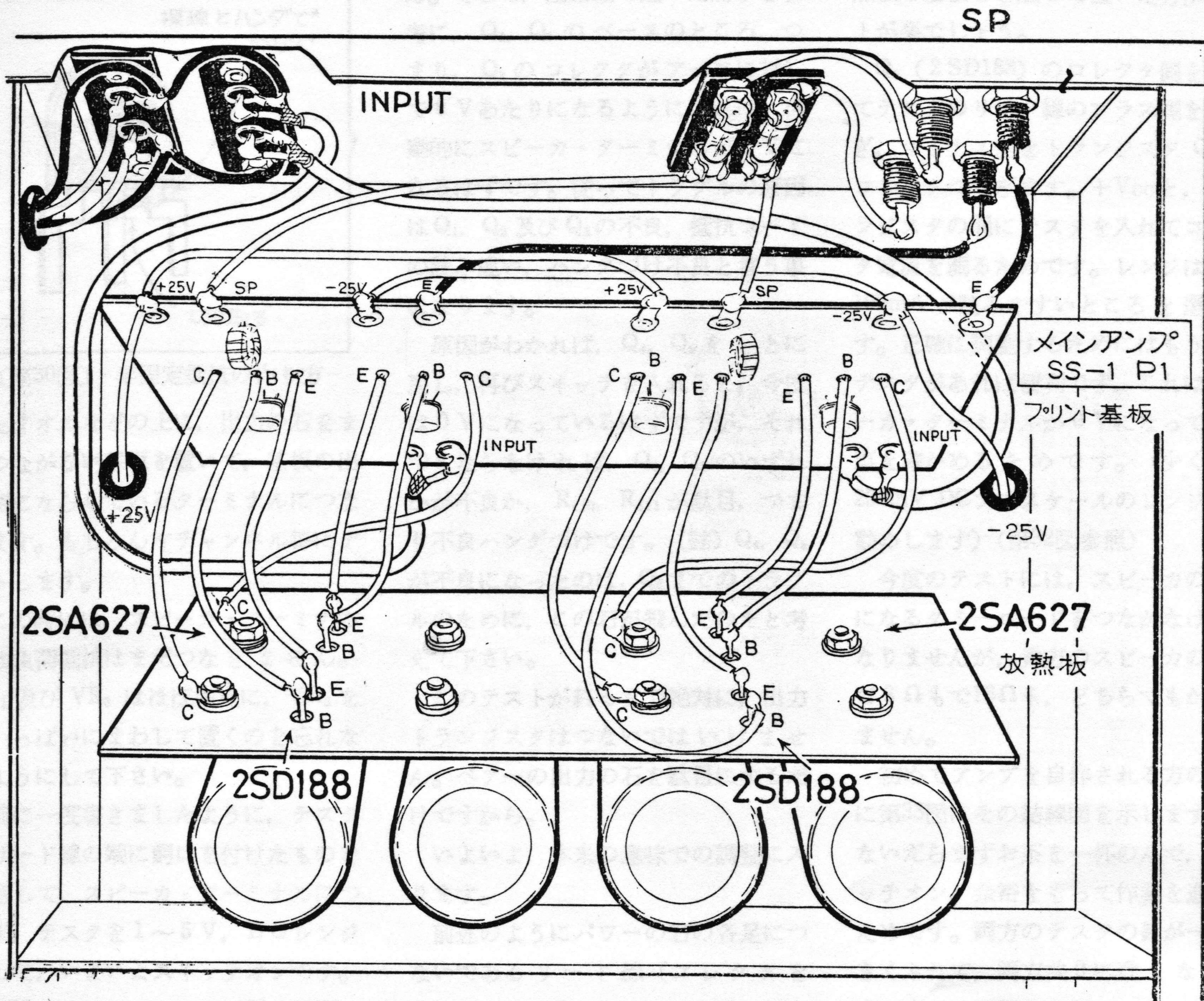
[メインアンプ部の実体図]
