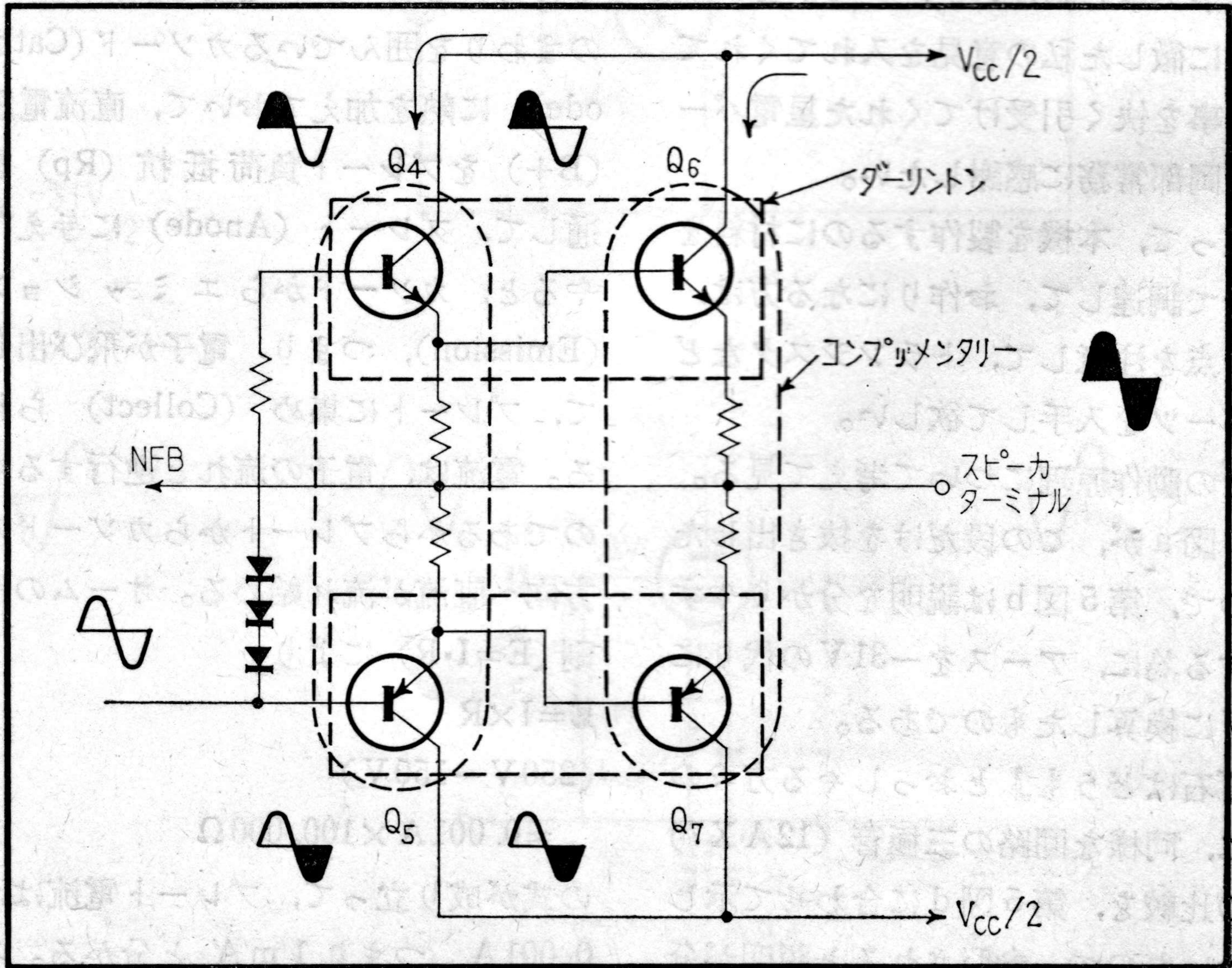
〔第7図〕出力段
