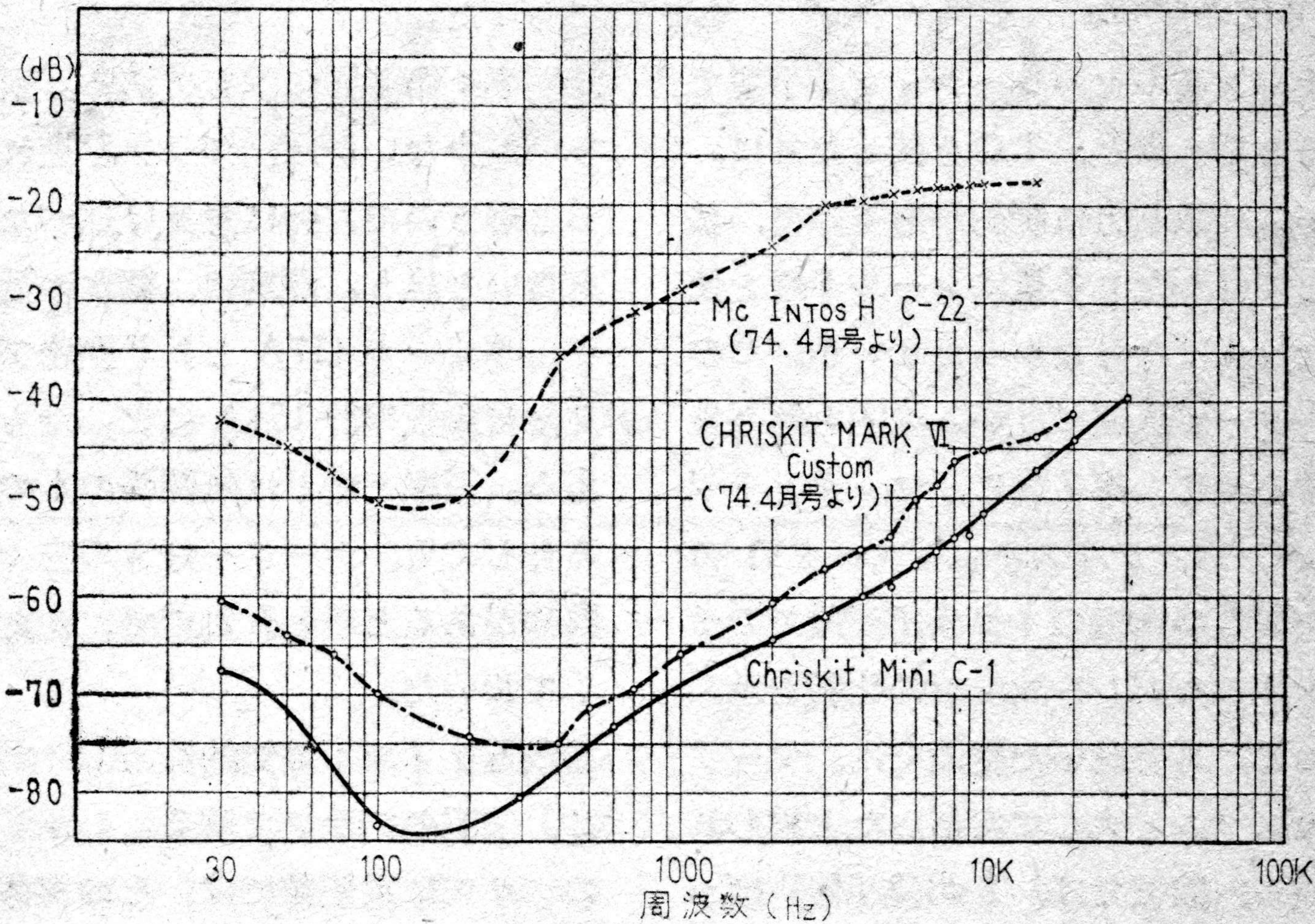
〔第7図〕 マッキントッシュC-22, クリスキットマークVIカスタム及び本機のイコライザ段でのチャンネルセパレーションの比較
