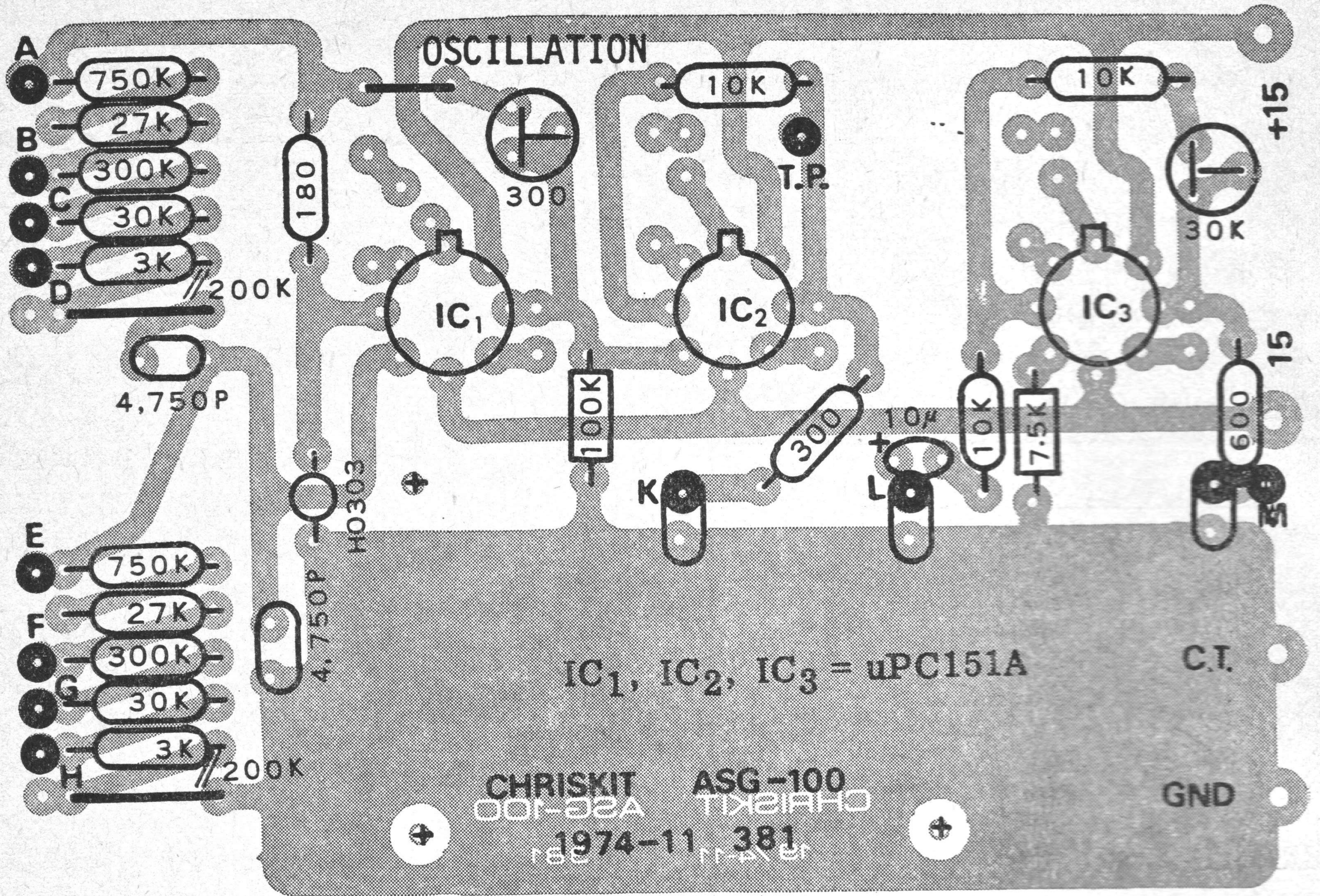
〔第7図〕 プリント基板のパターン及び部品配置
