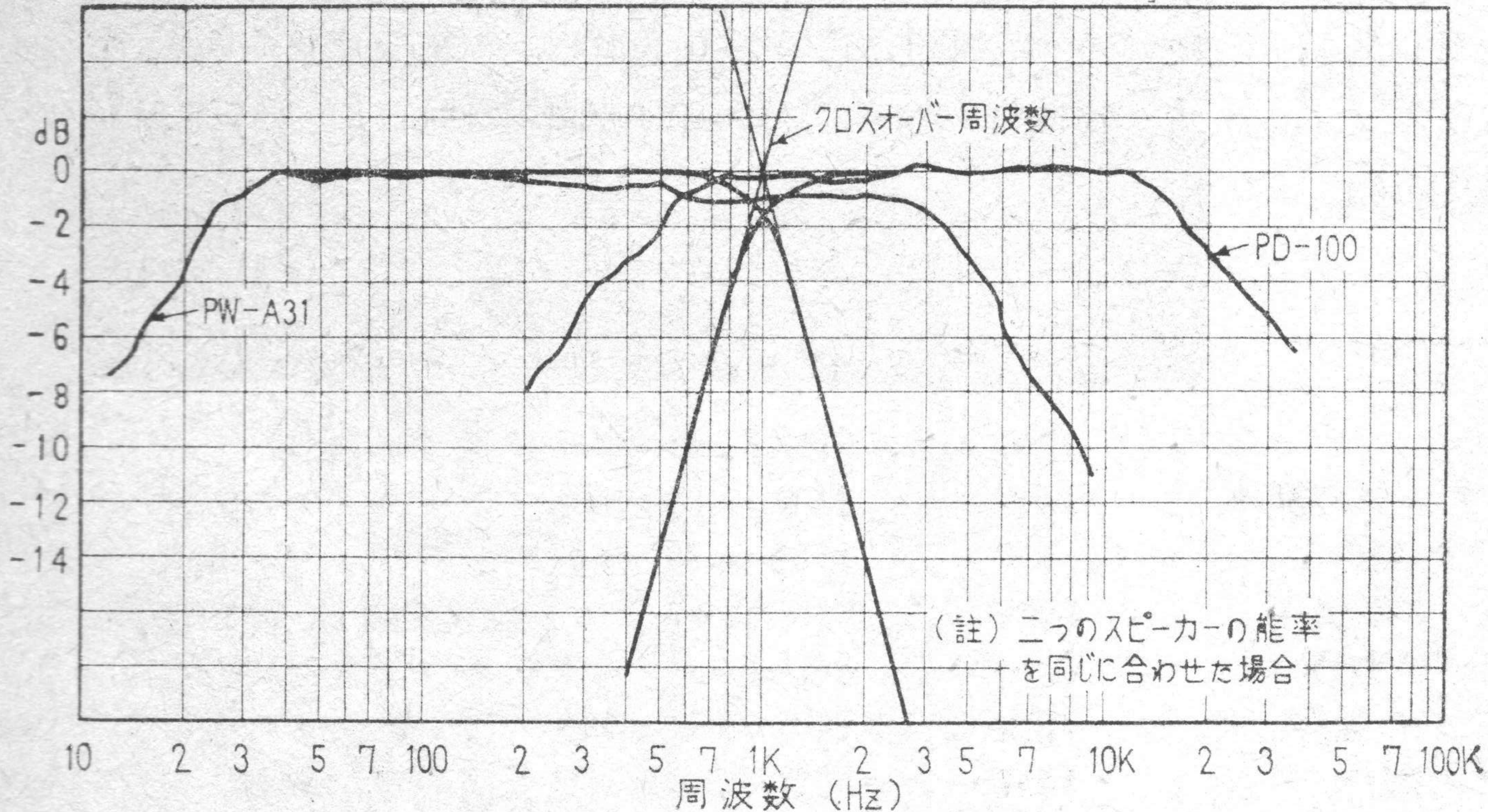
〔第51図〕 PD-100 及び PW-A31 周波数特性
