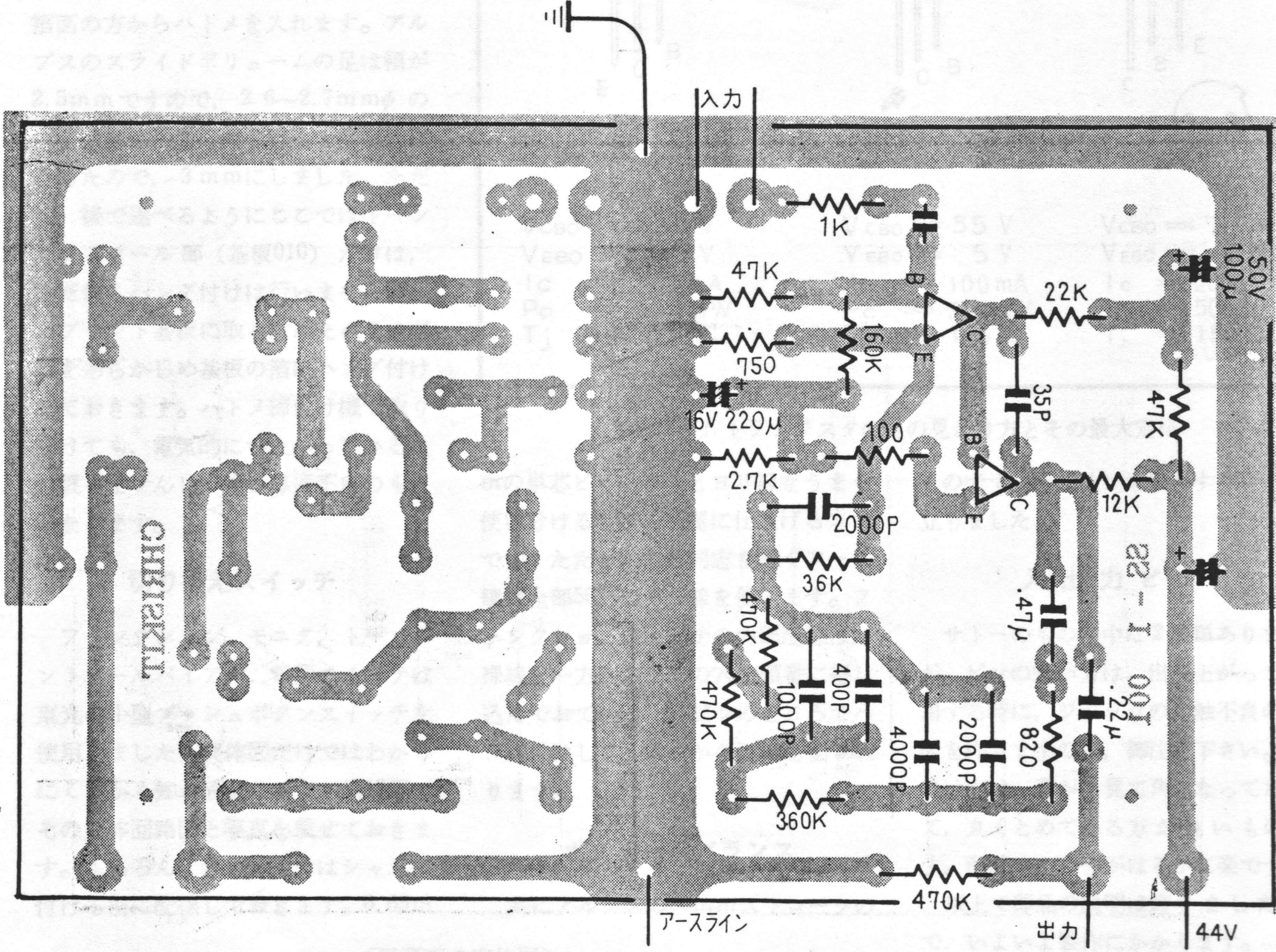
(d) フラットアンプ部のパターン図 (左右チャンネル対称)
