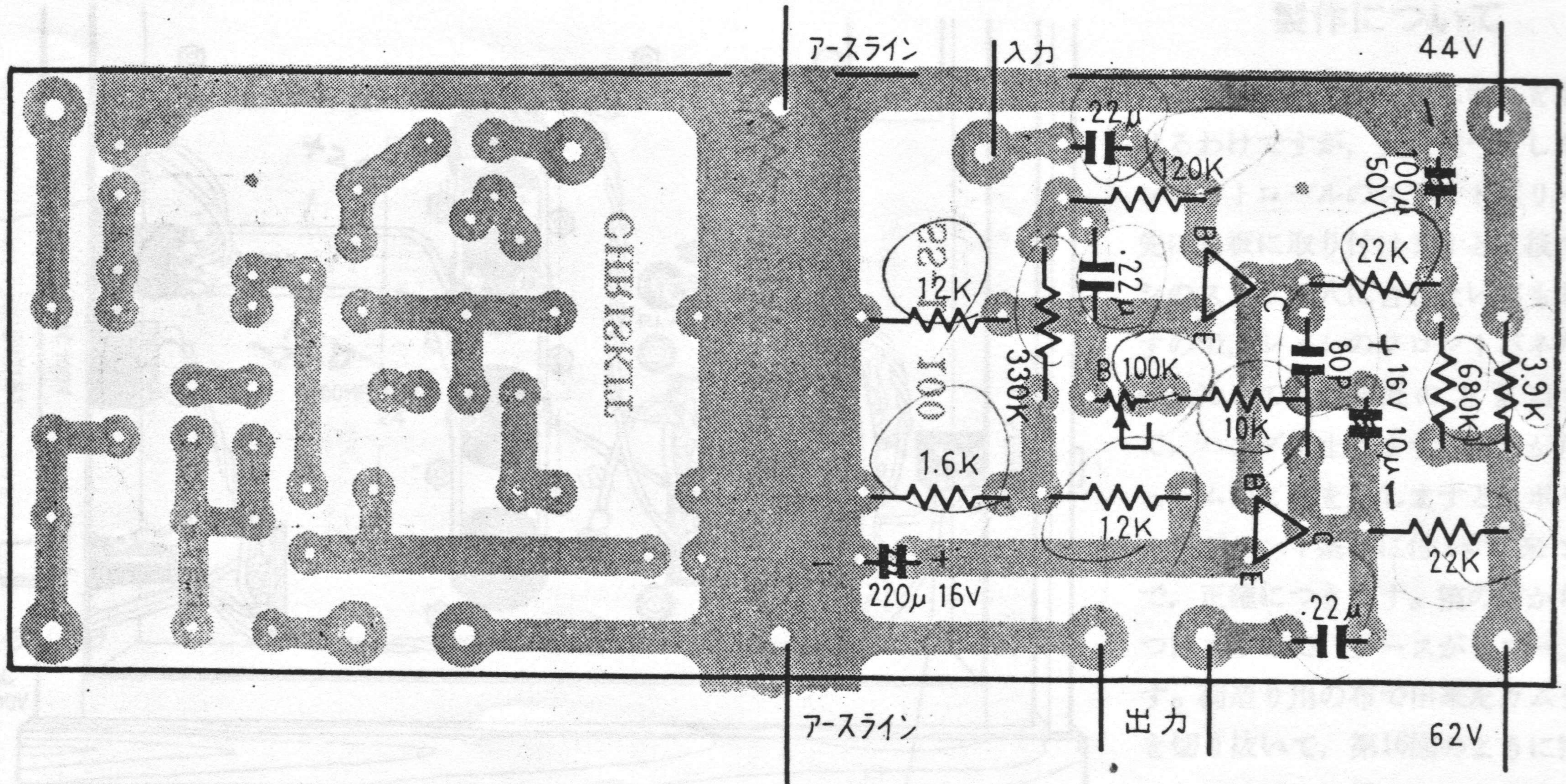
(d) フラットアンプ部のパターン図 (左右チャンネル対称)
