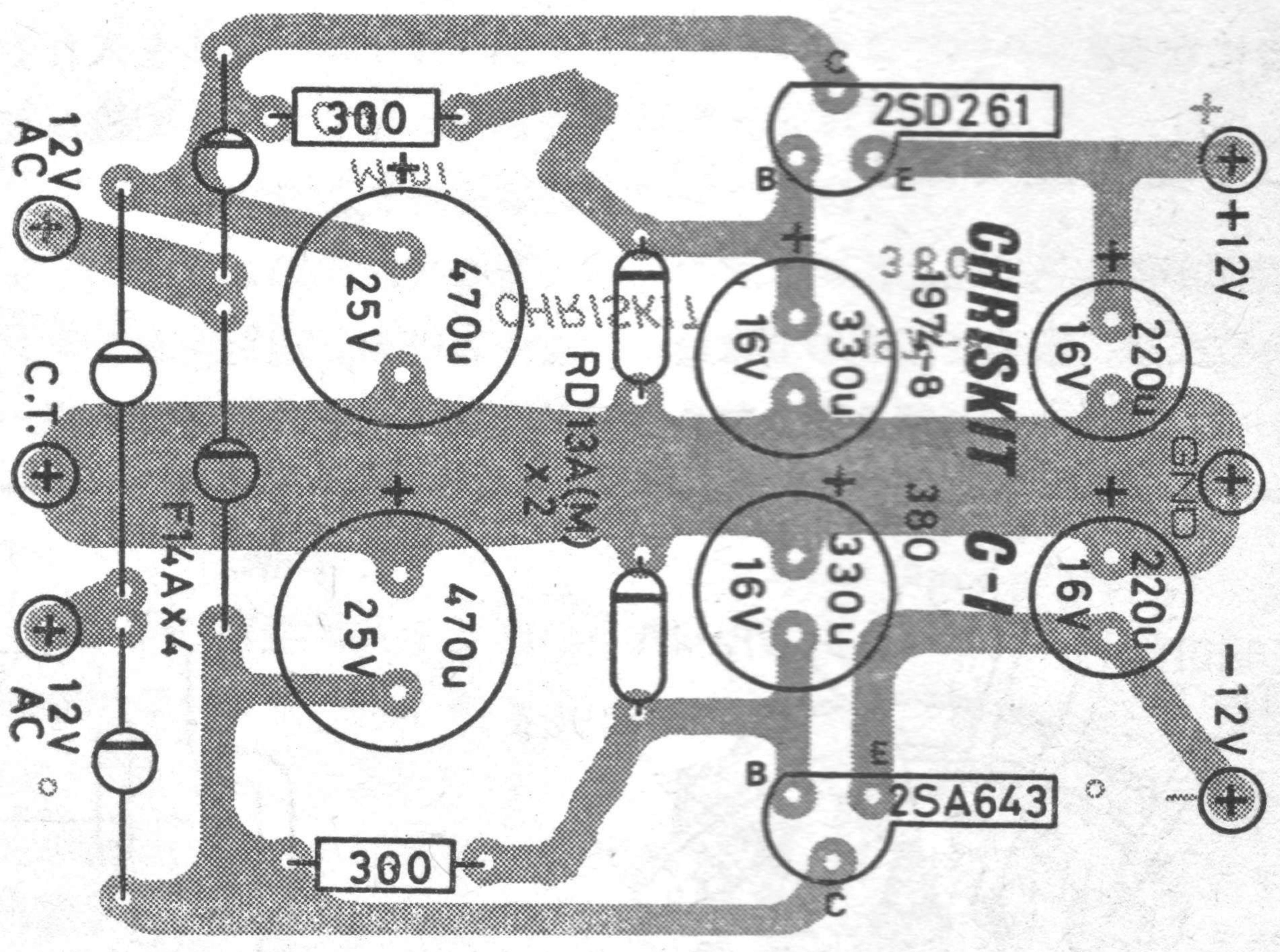
〔第3図〕プリント基板のパターン及び部品配置図
