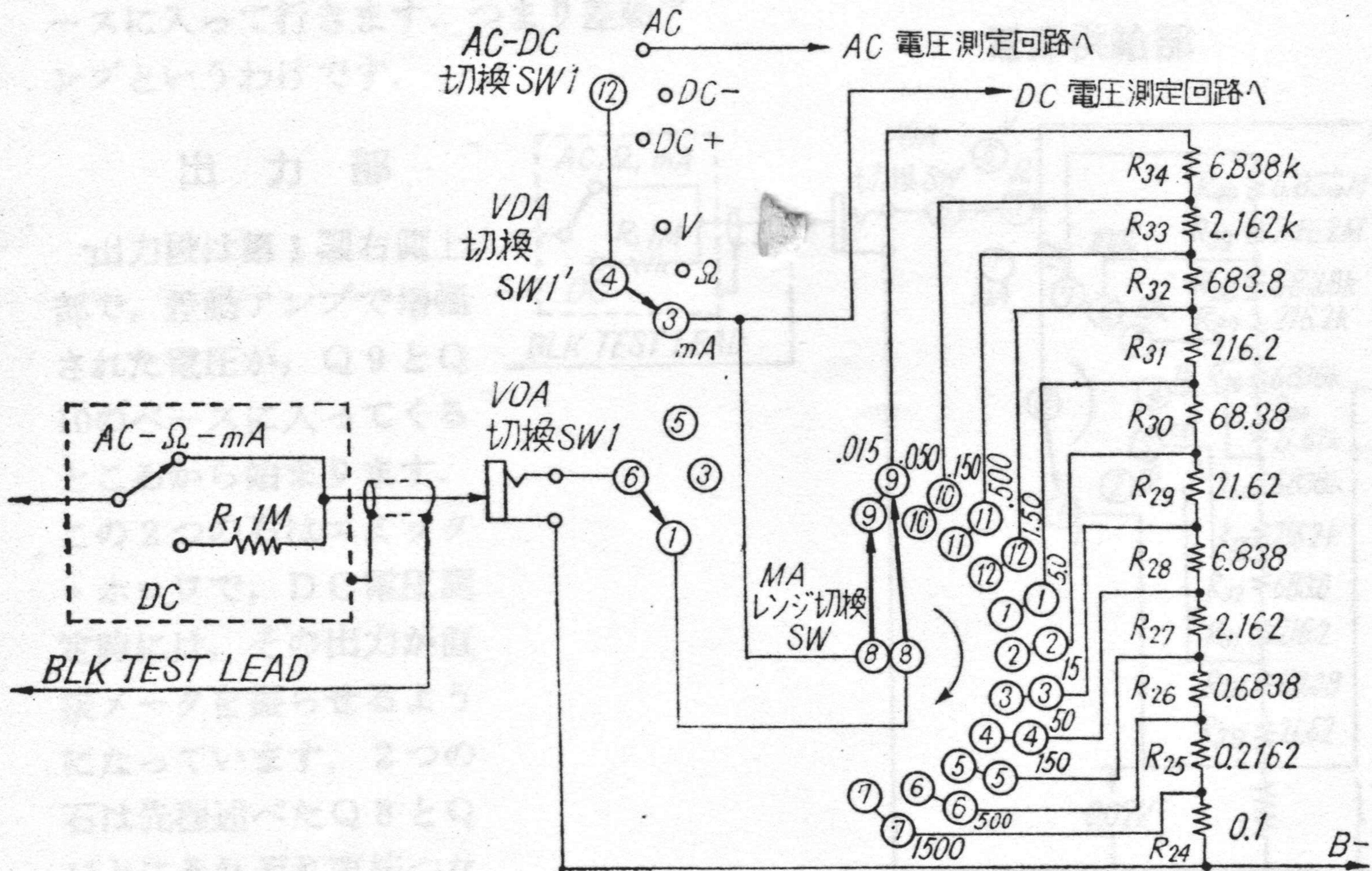
〈第3図〉 mA測定回路図
