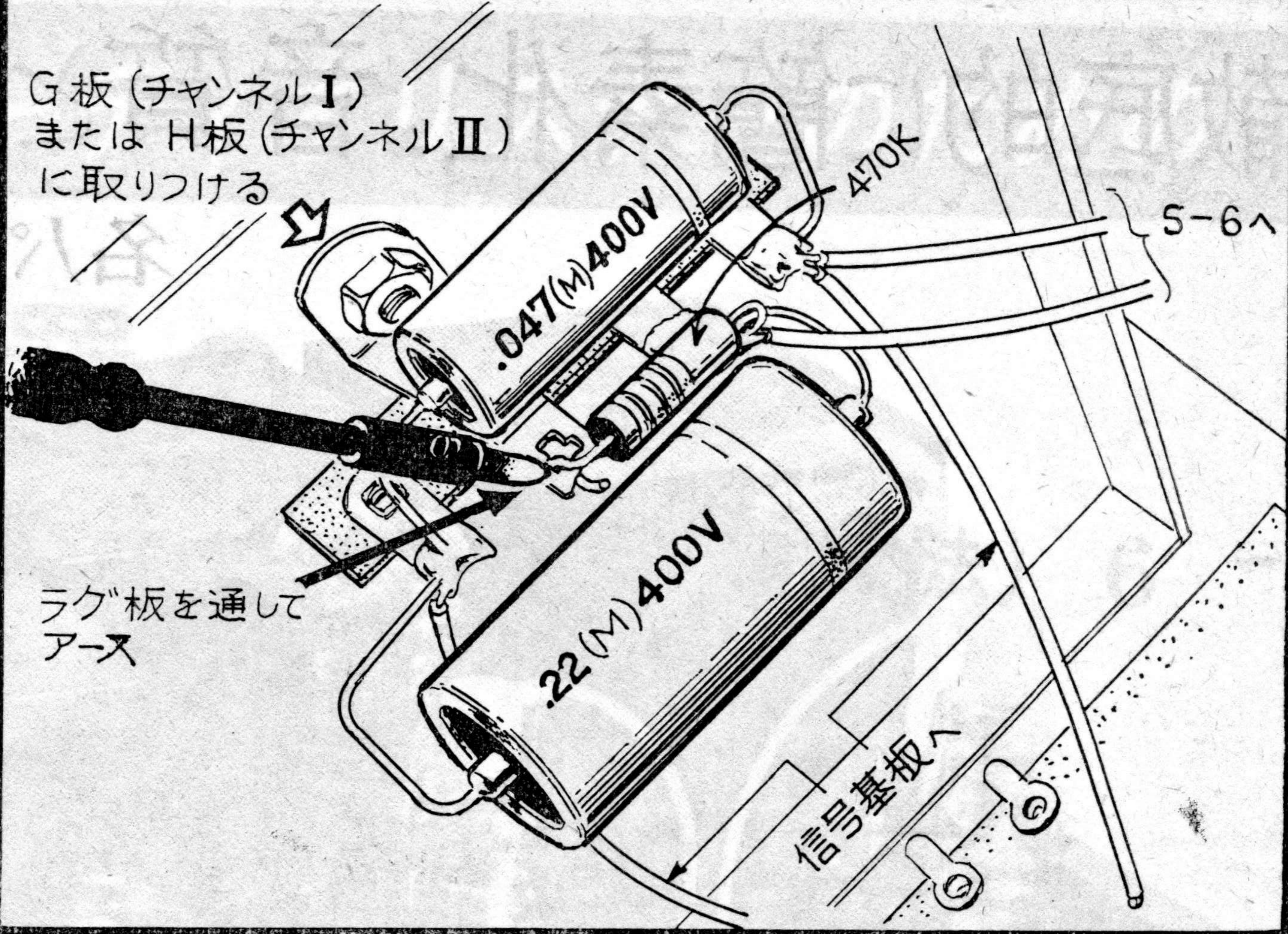
〔第21図〕 出力コンデンサ切換部の配線
