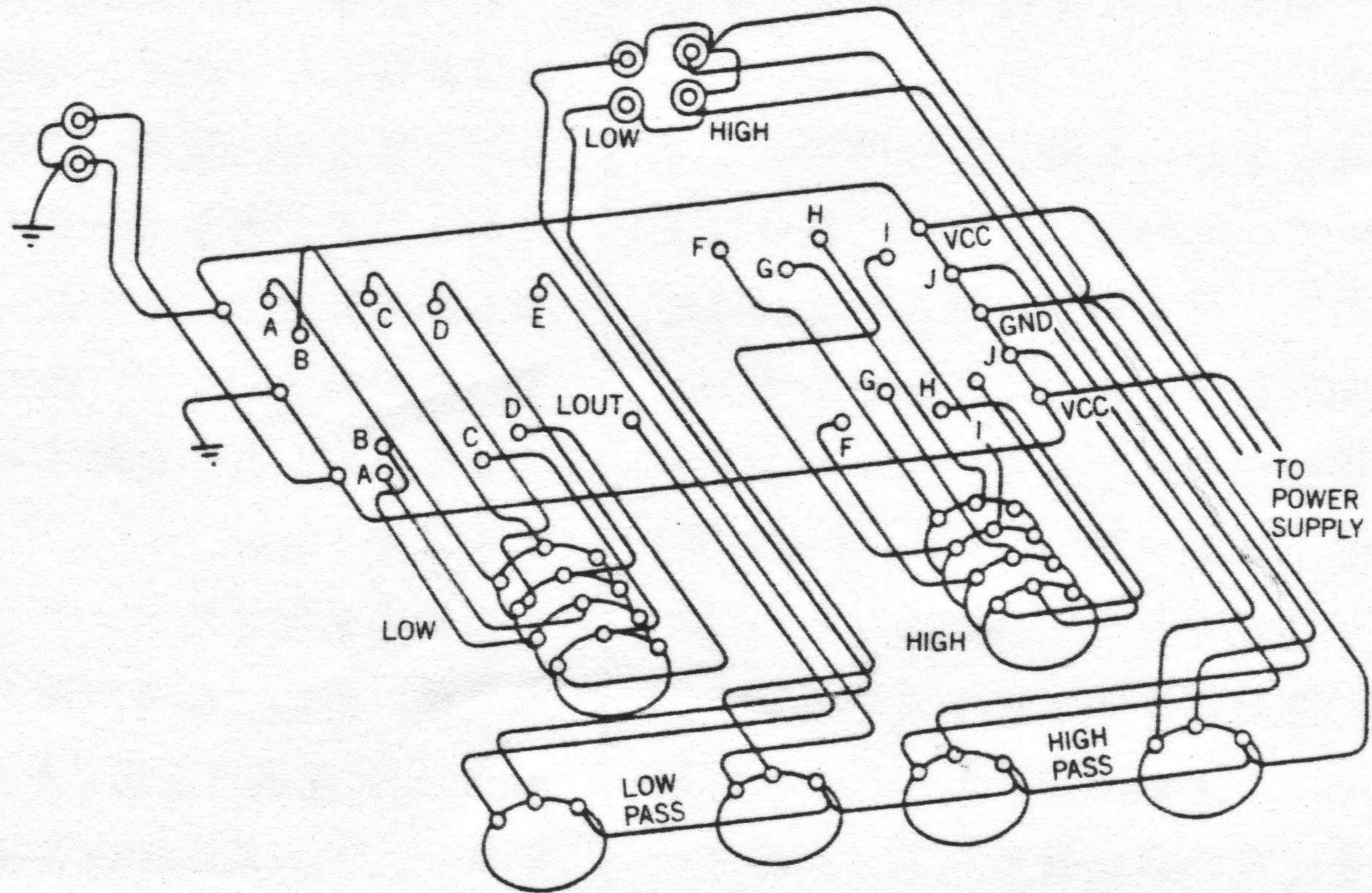
本機の実体回路図
