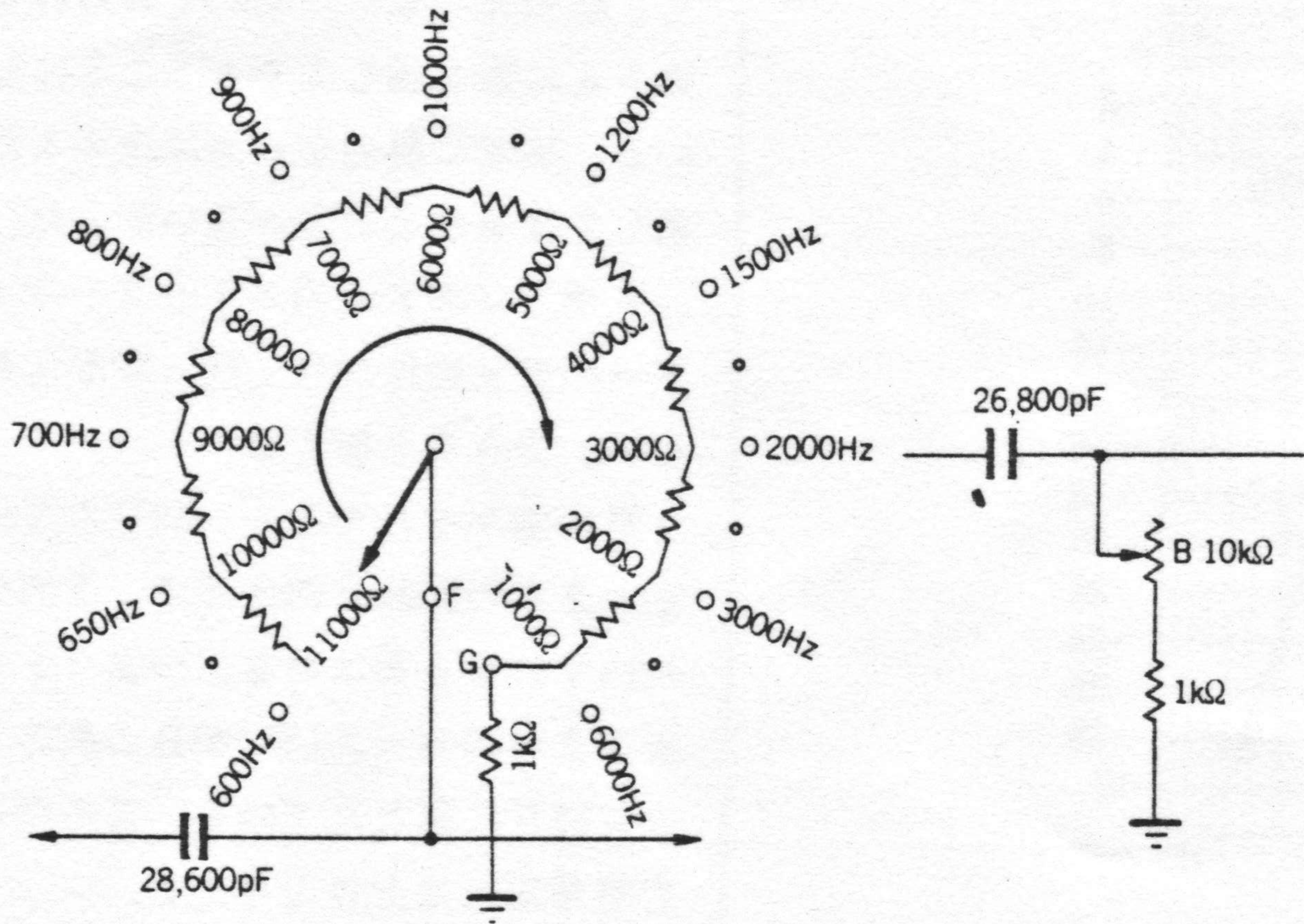
《第15図》 ハイパスフィルターの抵抗値変化
