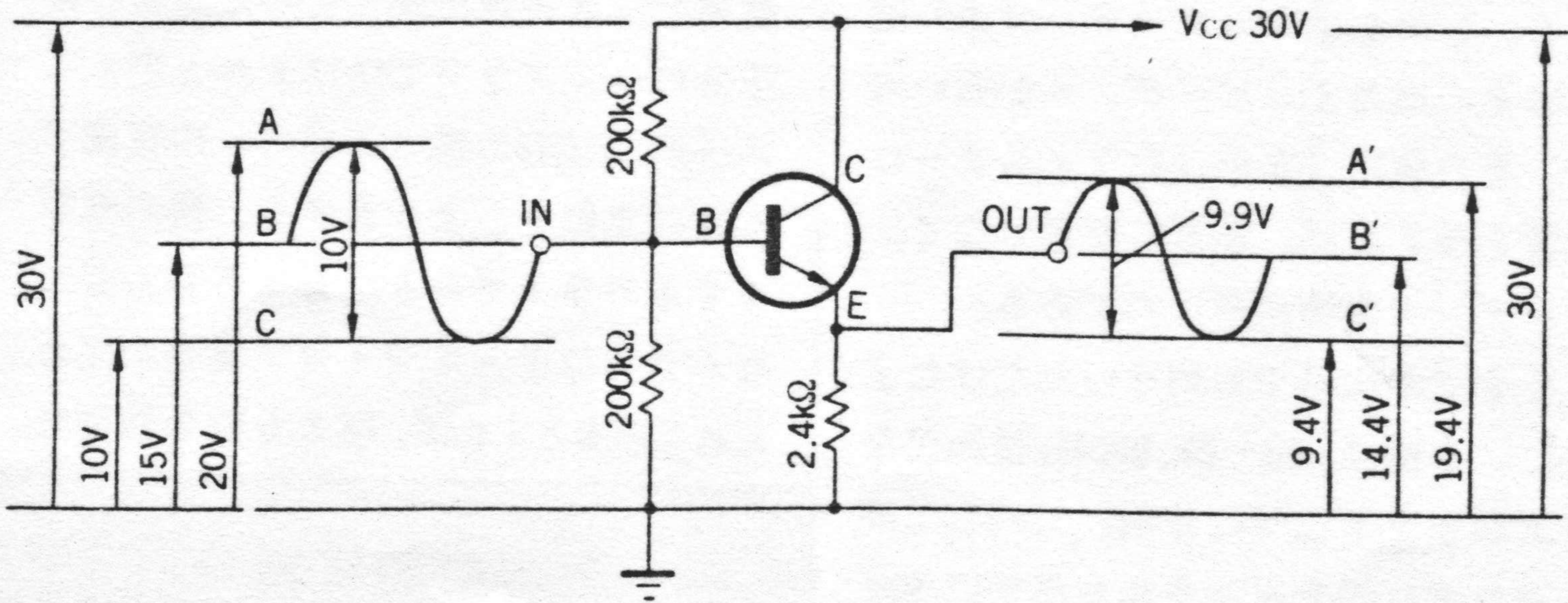
《第16図》 エミッターフォロアー回路
