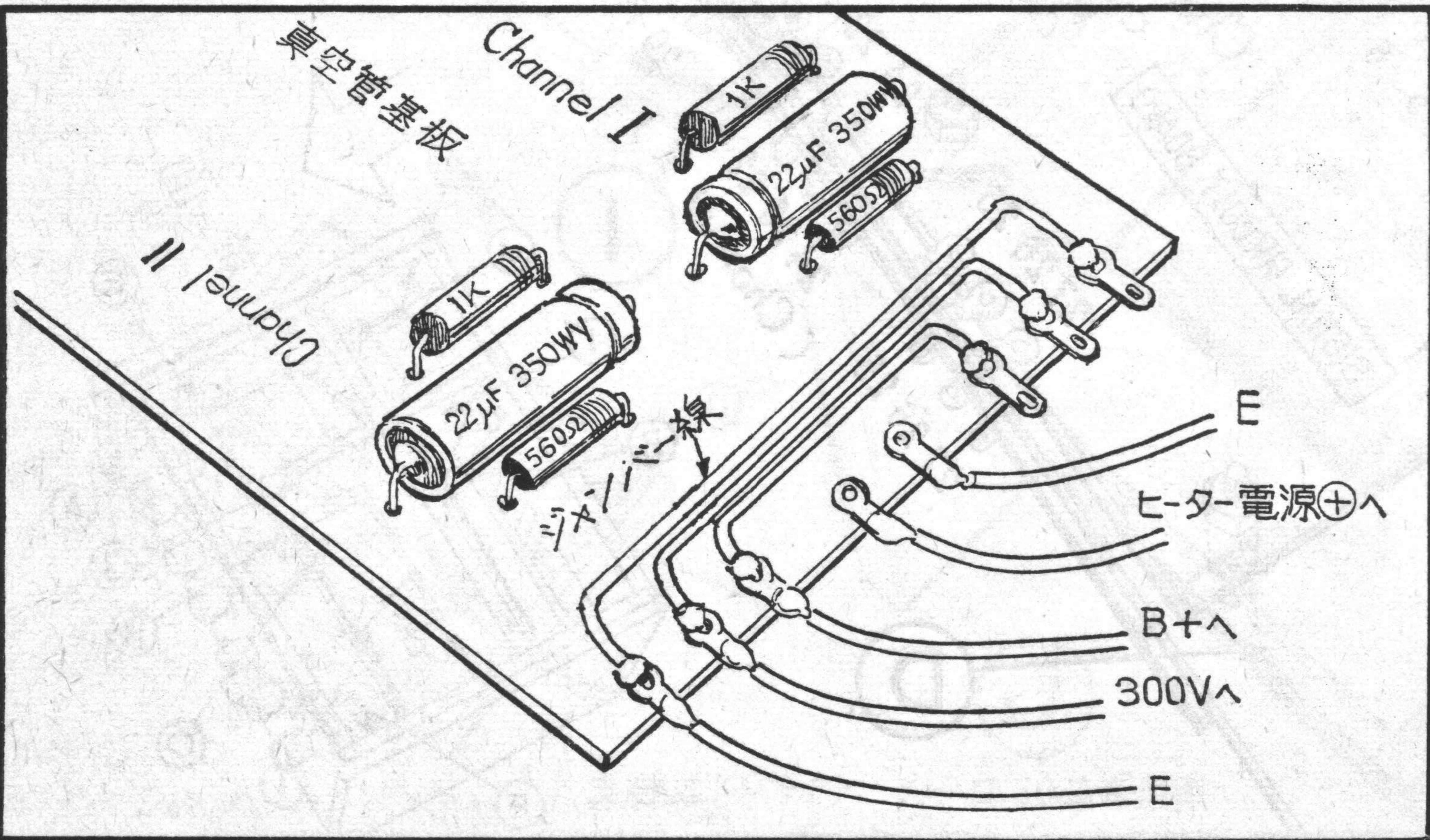
〔第18図〕 真空管基板の末端処理の方法
